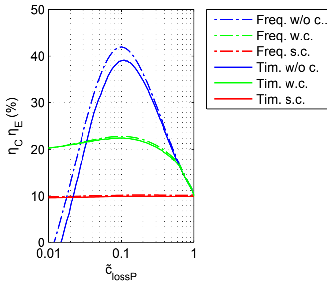
FIGURE 2.11 – Efficacité globale de la récupération \eta_C \eta_E dans le cas multichromatique ( H_s = 2.5 m, T_p = 9.5 s) en fonction du coefficient de pertes \tilde{c}_{loss P} pour le contrôle utilisé ( c_{loss P} = 0.1 ). Les couleurs correspondent aux contraintes liées à la stabilité : en bleu, pas de contraintes, en vert, contrainte faible et en rouge contrainte forte. Les traits continus correspondent aux résultats des simulations temporelles et les traits discontinus aux résultats attendus à partir de l'optimisation fréquentielle.
