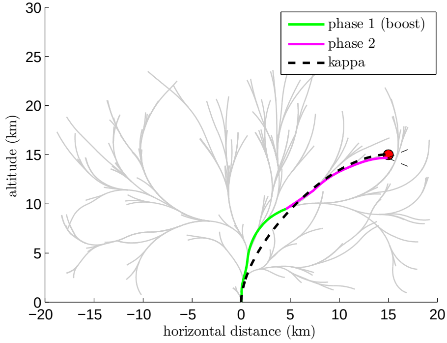
(a) \text{RRT}_{\text{kappa}} : Trajectories
