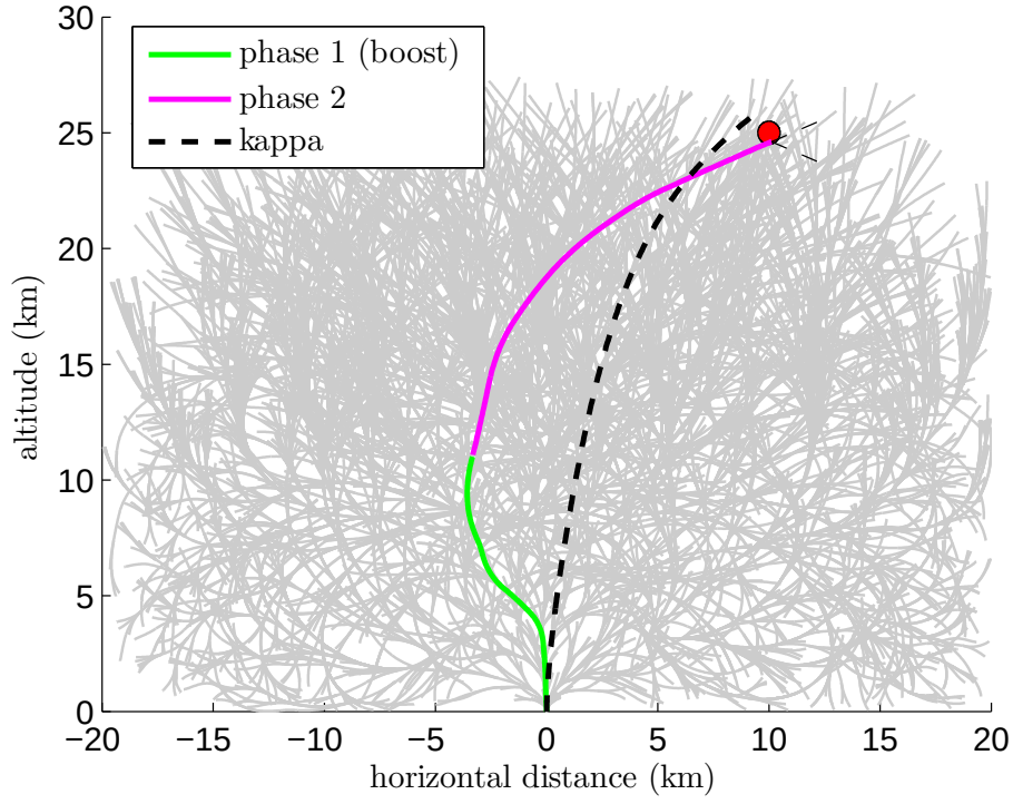
(a) \text{RRT}_{\text{kappa}} : Trajectories
