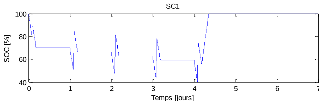
Figure 5.3 : Variation du SOC pendant une semaine typique avec le scénario SC1
