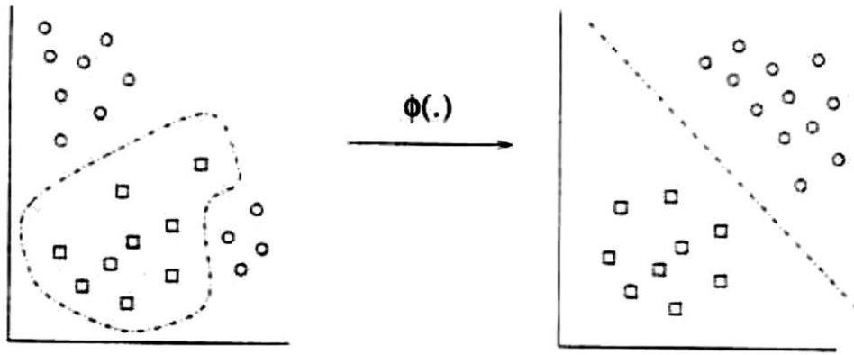
Fig. II : Projection des entrées dans un hyperplan de plus grande dimension, à l'aide de la fonction \Phi(.) , pour se ramener au cas linéaire
