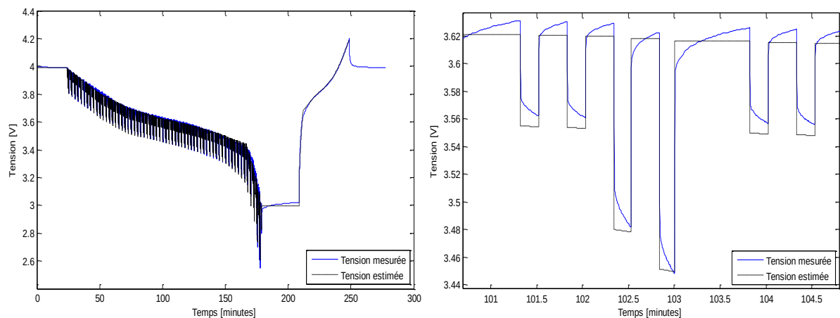
Figure 4.9 : Comparaison entre la tension mesurée et celle estimée : (a) sur toute la plage de SOC (b) zoom sur quelques créneaux de courant
