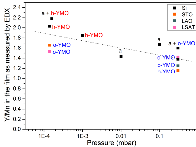
Figure R.7. La formation des phases en fonction de la pression d'O 2 et le rapport atomique Y/Mn dans les films déposés par PLD sur différents substrats à 800 °C.
