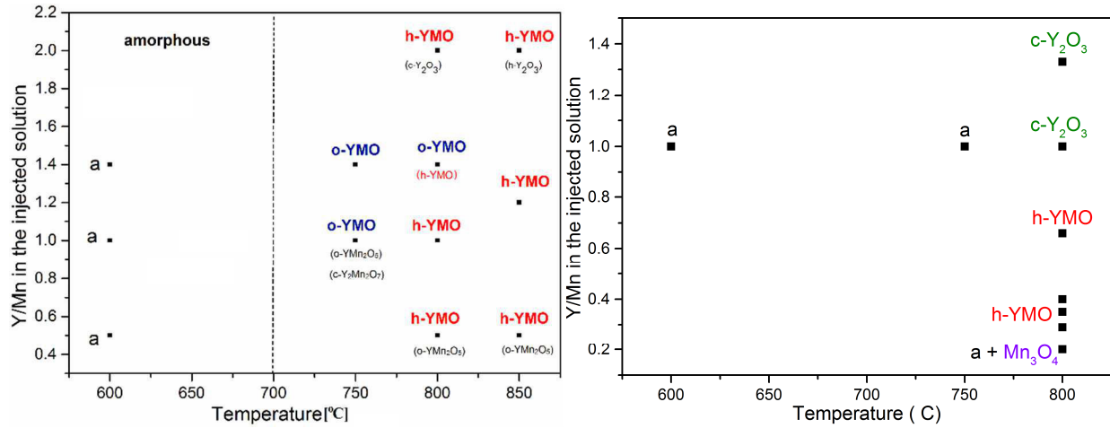
Figure R.6. Dépendance de la structure cristalline en fonction de la température et le rapport Y/Mn dans la solution injectée pour le réacteur PI-MOCVD vertical (a) et horizontal (b).
