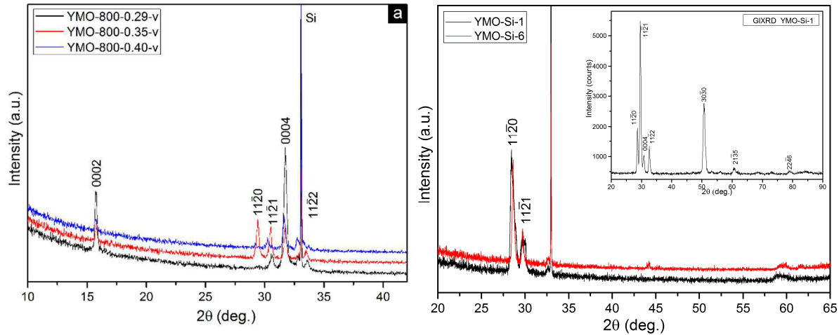
Figure R.9. a) Diagrammes XRD de films YMO indexés avec la phase h-YMO (JCPDS card No. 11-9577); b) les diffractogrammes XRD \theta - 2\theta de films h-YMO déposés par PLD à différentes pressions d'O 2 . En encadré: Le GIXRD de l'échantillon YMO-Si-1.
