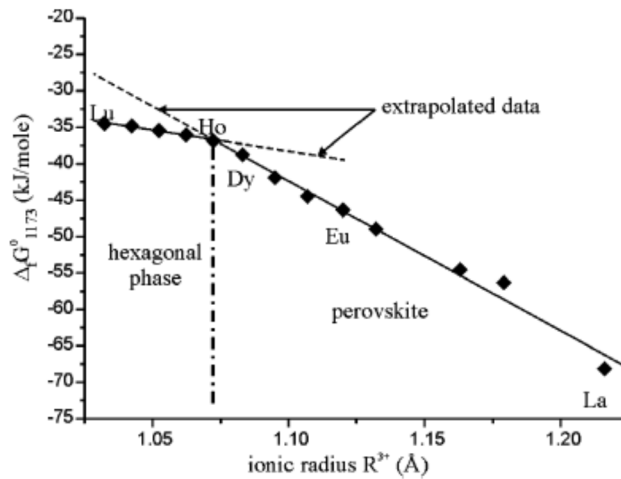
Figure R.5. L'énergie libre de formation de Gibbs de RMnO_3 à partir de R_2O_3 et Mn_2O_3 à 900\text{ °C} et à la pression ambiante ([10]).
