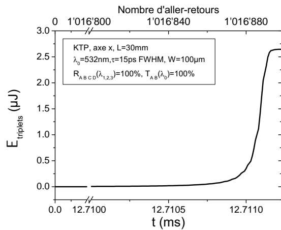
(b) Energie de triplets générée en fonction du temps (ou du nombre d'aller-retours), pour une propagation dans un TROPO de KTP de longueur 30 mm et pour une énergie initiale de pompe de E_0 = 1 \mu\text{J} .
