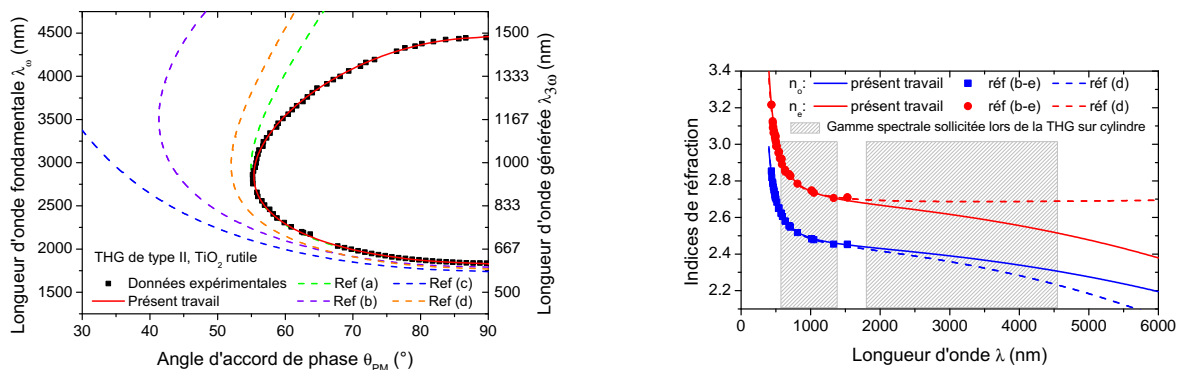
(a) Courbe d'accord de phase de THG de type II du \text{TiO}_2 rutile. Les données expérimentales de l'expérience du cylindre sont représentées en carrés noirs, et leur interpolation numérique est la courbe rouge. Les courbes d'accord de phase en pointillés sont calculées à partir de données bibliographiques.
