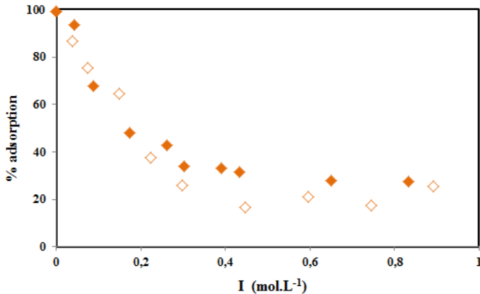
Figure IV.5: effet de la force ionique I sur l'adsorption de méthylorange par les billes de chitosane \blacklozenge NaCl; \diamond CaCl 2 ; C_0=0,301\pm0,002 mmol.L -1 ( 0,049\pm0,001 mmol.g -1 ; 98,9\pm0,2 mg.L -1 ); m_b= 2,15\pm0,01 g; V=20 mL; pH\approx 4 .
