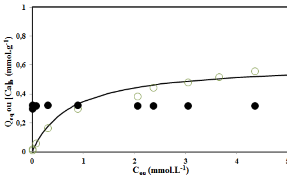
Figure VI.9: isotherme d'adsorption du PNP par les billes AA 2 ; Q_{eq} (○) et [Ca]_b (●) ; Trait plein : modélisation par l'équation de Langmuir ; pH=6,0±0,6 ; t=2 jours ; m_b=0,533±0,004 g ; V=5 mL.
