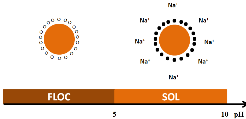
Figure II.10: effet du pH sur la stabilité d'un ferrofluide à base de nanoparticules fonctionnalisées par des ions citrate (○ \text{COOH} et ● \text{COO}^- ).
