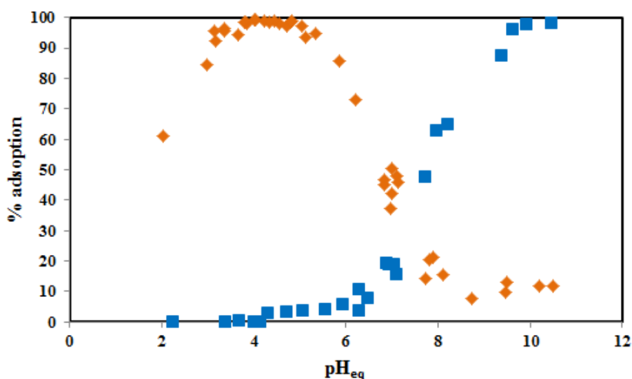
Figure IV.6: effet du pH sur l'adsorption du méthylorange et du bleu de méthylène par les billes de chitosane ( m_b=2,2\pm 0,1 \text{ g} ; V=20\text{mL} ; t= 2 \text{ jours} ): ◆ MO: C_0=0,216\pm 0,001 \text{ mmol.L}^{-1} ( 0,045\pm 0,001 \text{ mmol.g}^{-1} ; 70,8\pm 0,3 \text{ mg.L}^{-1} ); ■ BM: C_0=0,266\pm 0,001 \text{ mmol.L}^{-1} ( 0,042\pm 0,001 \text{ mmol.g}^{-1} ; 99,6\pm 0,2 \text{ mg.L}^{-1} ).
