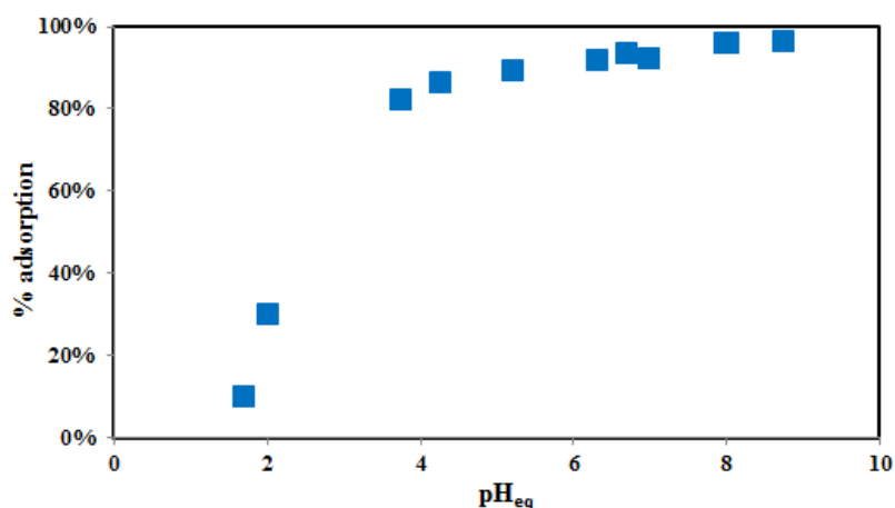
Figure IV.8: effet du pH sur l'adsorption du bleu de méthylène par les billes d'alginate ; C_0=0,3\text{mmol.L}^{-1} ( 0,05\text{mmol.g}^{-1} , 99,7\text{mg.L}^{-1} ) ; m_b=2,149\pm 0,004\text{g} , V=20\text{mL} , t=2\text{jours} .
