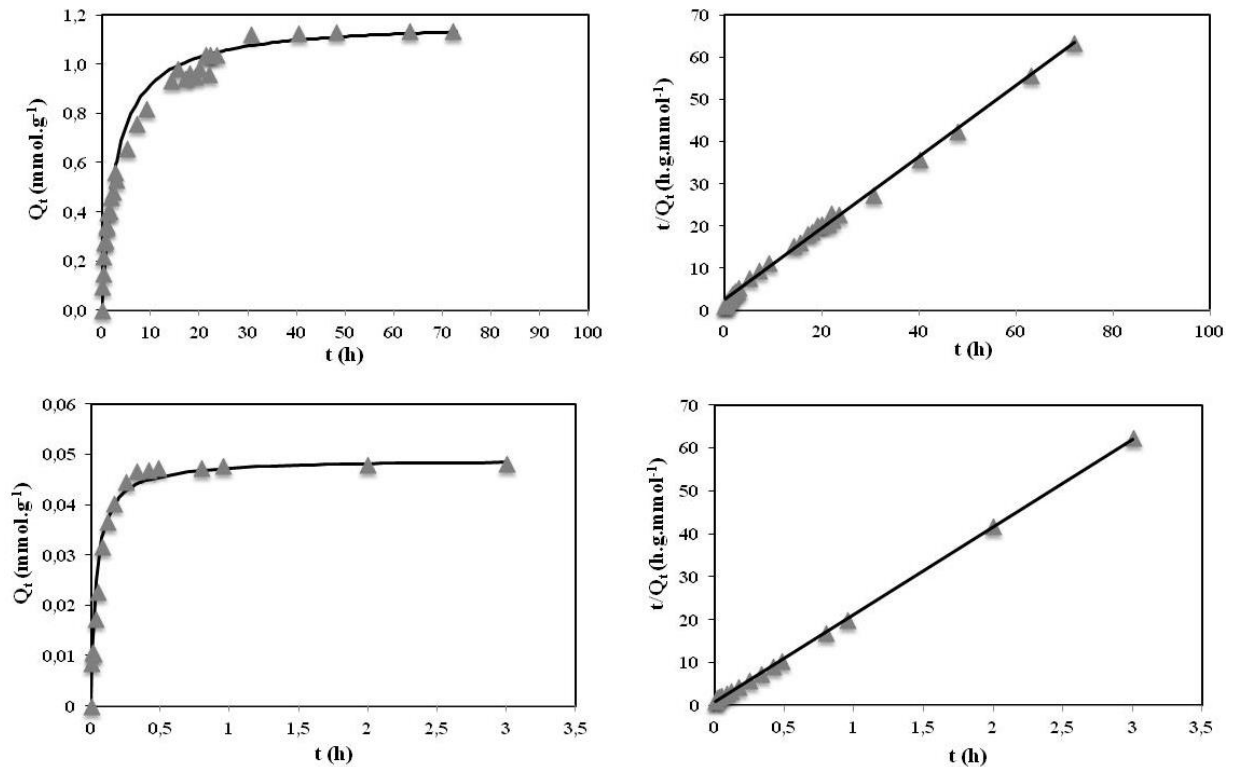
Figure V.12: modélisation de la cinétique d'adsorption du CPC par une équation pseudo-ordre 2 : (haut) C_0=1,15±0,01 mmol.g -1 ; (bas) C_0=0,0492±0,0002 mmol.g -1 .
