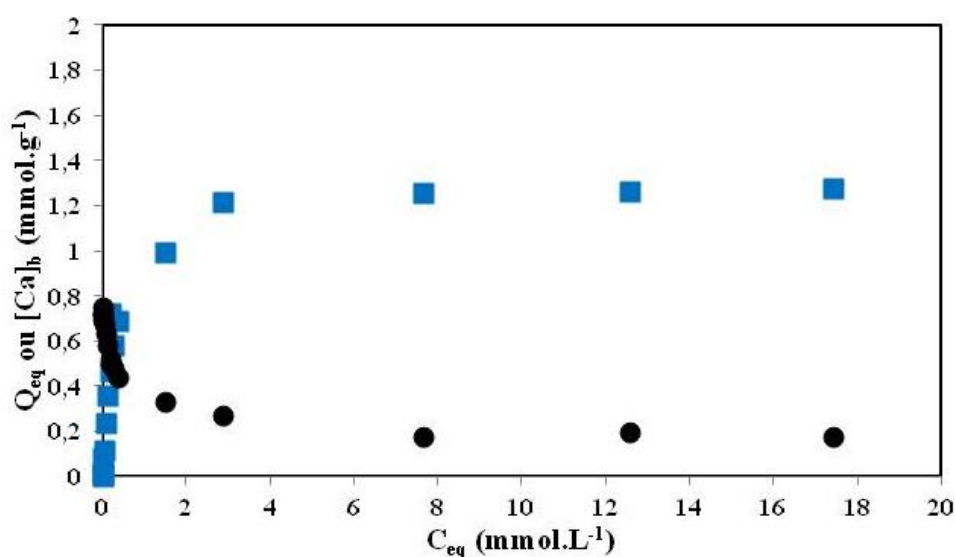
Figure V.10: isotherme d'adsorption du BM par les billes d'alginate magnétiques; Q_{eq} (■); [\text{Ca}]_b (●); m_b=2,149\pm 0,004 \text{ g} ; t=2 \text{ jours} ; pH_{eq}=6,8\pm 0,2 ; V=20 \text{ mL} .
