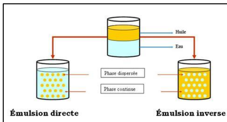
Figure 1: représentation schématique des émulsions inverse et directe
