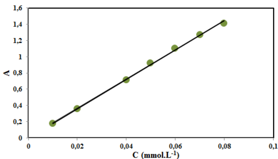
Figure II.8: droite d'étalonnage du p-nitrophénol effectuée à 259 nm.
