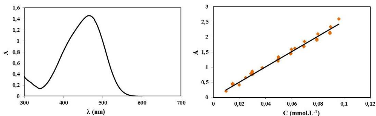
Figure II.3: spectre UV-visible (gauche) et droite d'étalonnage (droite) du méthylorange
