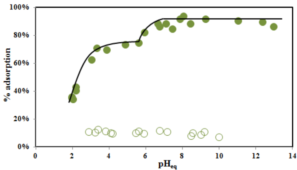
Figure V.23: PNP (%) adsorbé en fonction du pH ; ○ sans CPC ; C_{0,PNP}=0,111 \pm 0,012 \text{ mmol.g}^{-1} ; t=2h-24h ; ● avec CPC, C_{0,CPC}=1,20 \pm 0,03 \text{ mmol.g}^{-1} ; C_{0,PNP}=0,122 \pm 0,002 \text{ mmol.g}^{-1} , t=3 \text{ jours} . La ligne continue est un guide pour l'œil.
