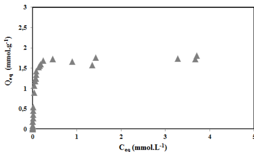
Figure V.6: isotherme d'adsorption du CPC par les billes d'alginate magnétiques; m_b \approx 2,15 \text{ g} ; V=20 \text{ mL} ; pH_{eq}=7,0 \pm 0,5 ; t=3 \text{ jours} .
