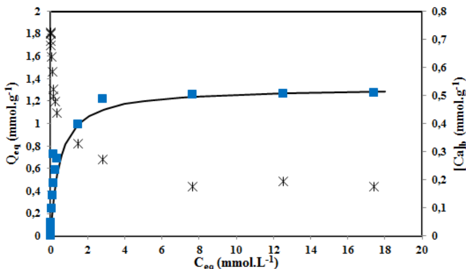
Figure IV.11: isotherme d'adsorption du bleu de méthylène par les billes d'alginate (■ Q_{eq} (mmol.g -1 ), axe de gauche) et évolution de la concentration en ions Ca 2+ dans les billes (* [Ca]_b (mmol.g -1 ), axe de droite).
