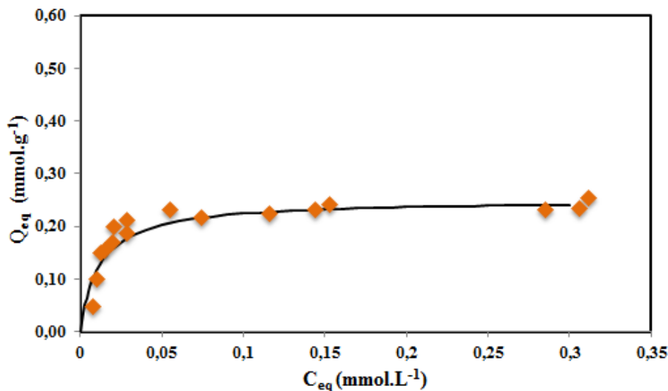
Figure II.19: isotherme d'adsorption du méthylorange par des nanoparticules de maghémite non fonctionnalisées; pH_{eq}=4,0\pm 0,1 ; m_{magh}=40 mg; V=20 mL; t\geq 20h . La courbe en trait plein est la courbe théorique obtenue à partir des paramètres de Langmuir.
