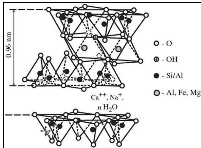
Figure VI.2: structure d'une montmorillonite [292] .
