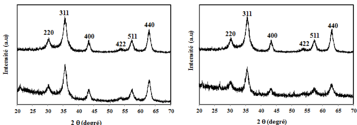
Figure III.12: diffractogramme des produits séchés ; à gauche : Billes magnétiques d'alginate (bas), \text{FF}_{\text{cit}} (haut) ; à droite : Billes magnétiques de chitosane (bas), \text{FF}_a (haut).
