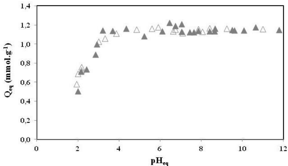
Figure V.22: effet du pH sur l'adsorption du CPC ; En absence de PNP (△), C_{0,CPC}=1,19 \pm 0,04 \text{ mmol.g}^{-1} ; En présence de PNP (▲), C_{0,PNP}=0,122 \pm 0,002 \text{ mmol.g}^{-1} , C_{0,CPC}=1,20 \pm 0,03 \text{ mmol.g}^{-1} .
