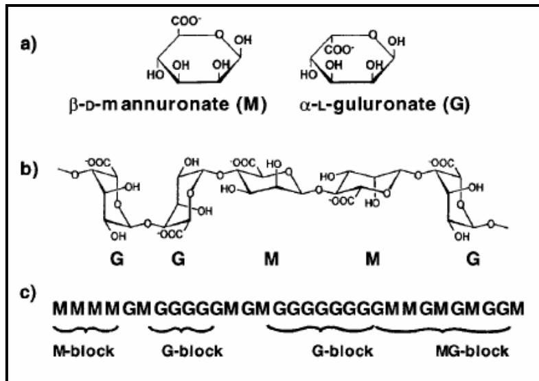
Figure III.1: présentation d'une structure d'alginate, (a) monomères mannuronate M et guluronate G ; (b) conformation des chaînes ; (c) exemple d'enchaînement des blocs M, blocs G et blocs alternés MG dans une chaîne d'alginate [158] .
