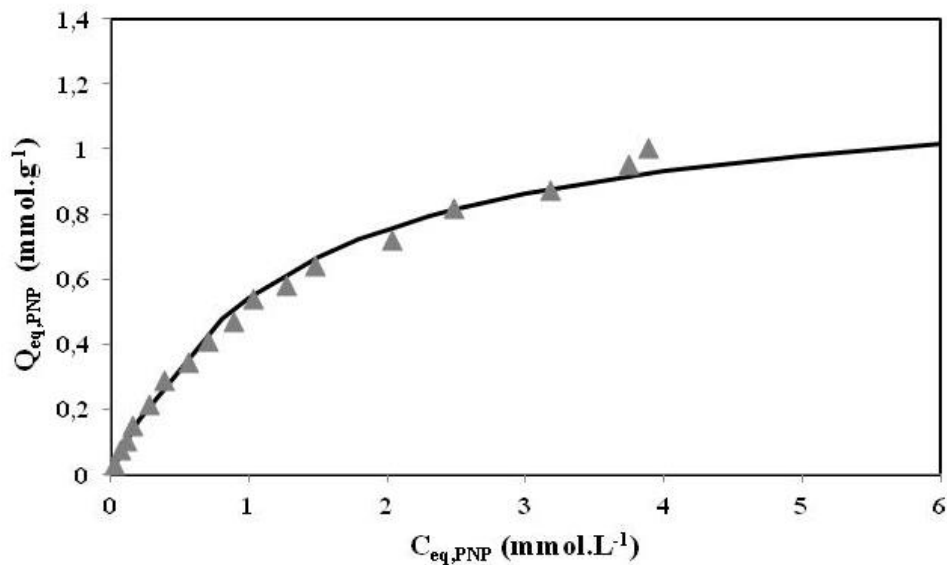
Figure V.18: isotherme d'adsorption du PNP; C_{0,CPC} = 1,16 \pm 0,01 \text{ mmol.g}^{-1} ( 6,76 \pm 0,12 \text{ mmol.L}^{-1} ); m_b \approx 1,075 \text{ g} ; V = 10 \text{ mL} ; t = 3 \text{ jours} ; Train plein : modélisation par l'équation de Langmuir.
