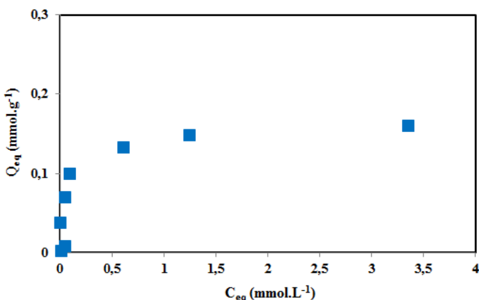
Figure IV.7: isotherme d'adsorption du bleu de méthylène ; m_b = 1,076 \pm 0,005 g ; V = 10 mL ; pH = 9,9 \pm 0,4 ; t = 2 jours.
