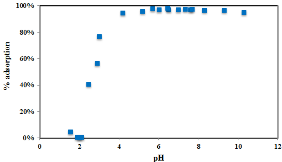
Figure II.15: effet du pH sur l'adsorption du bleu de méthylène par les nanoparticules citratées ; C_0=0,39 \text{ mmol.L}^{-1} ( 0,207 \text{ mmol.g}_{\text{magh}}^{-1} ; 146 \text{ mg.L}^{-1} ) ; t>24 \text{ heures} ; V \approx 20 \text{ mL} ; m_{\text{magh}}=38,6 \text{ mg} .
