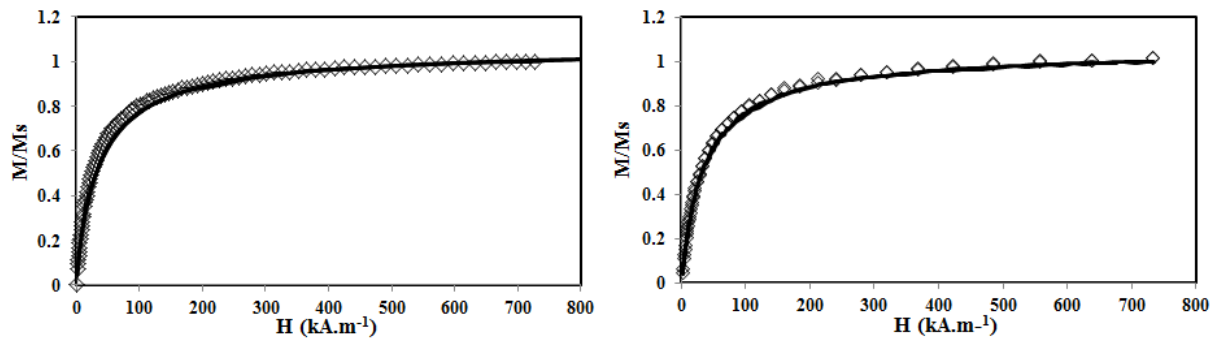
Figure III.13: courbes d'aimantation des billes et des ferrofluides normalisées par l'aimantation à saturation; billes d'alginate (gauche) ; billes de chitosane (droite). La ligne continue représente la courbe d'aimantation normalisée du ferrofluide ( FF_{cit} : gauche ; FF_a : droite).
