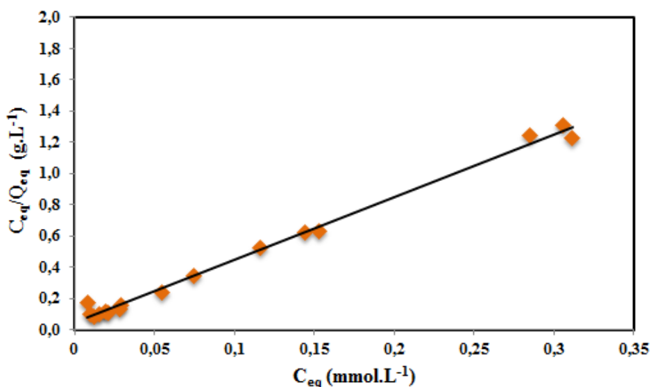
Figure II.20: linéarisation selon le modèle de Langmuir de l'isotherme d'adsorption du méthylorange par des nanoparticules magnétiques non fonctionnalisées.
