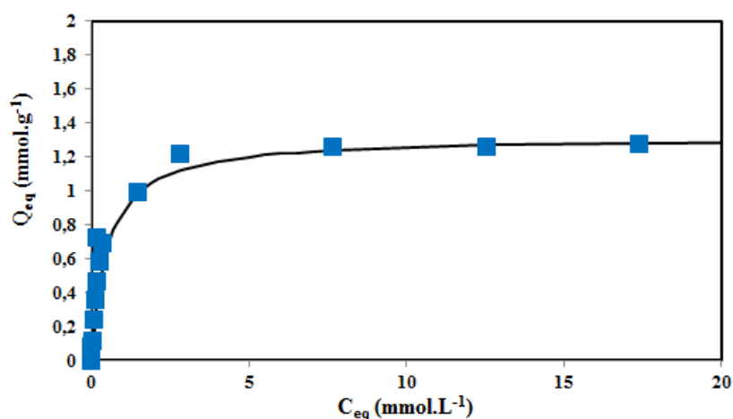
Figure IV.9: isotherme d'adsorption du bleu de méthylène par les billes d'alginate; m_b=2,149\pm 0,004 g, t=2 jours ; pH_{eq}=6,8\pm 0,2 ; V=20 mL ; Train plein : modélisation par l'équation de Langmuir.
