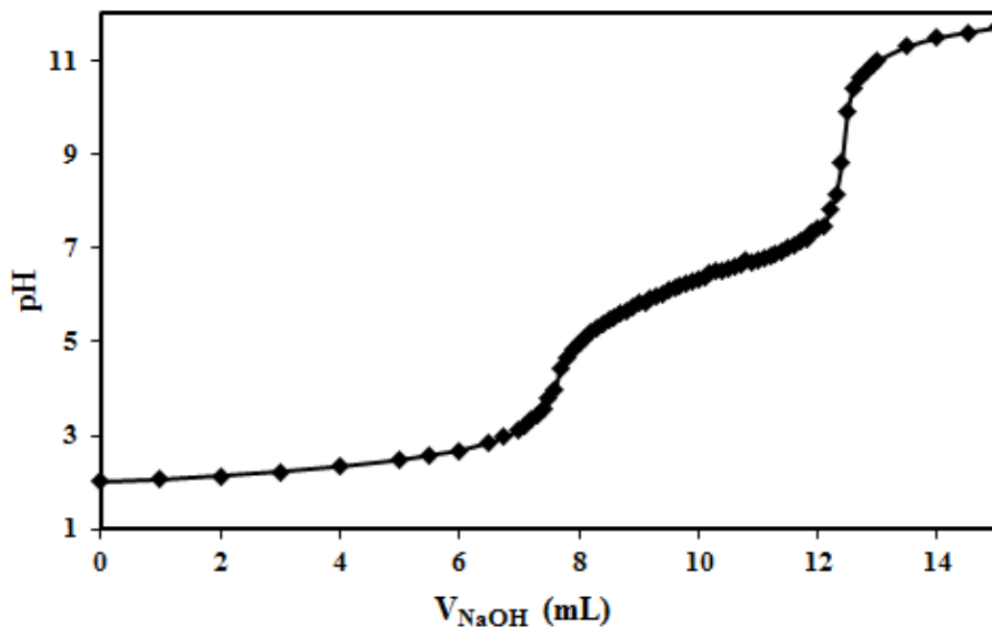
Figure III.4: exemple de dosage potentiométrique par la soude d'une solution de chitosane dissous dans un excès d'acide chlorhydrique ; m_{CH}=0,1055\text{ g} ; V_{HCl}= 1,2\text{ mL} ; C_{HCl}=1\text{ mol.L}^{-1} ; C_{NaOH}=0,1\text{ mol.L}^{-1} .
