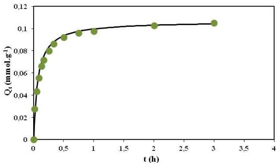
Figure V.29: cinétique d'adsorption du PNP par les billes d'alginate (Méthode 2); C_{0,PNP}=0,123\pm 0,001 mmol.g -1 ; C_{0,CPC}=1,282\pm 0,006 mmol.g -1 ; pH=6,5\pm 0,2 .
