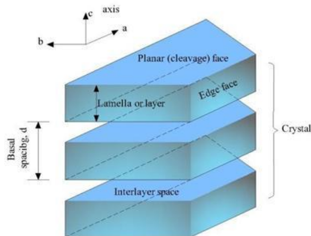
Figure VI.1: structure générale de la particule primaire des phyllosilicates [288] .
