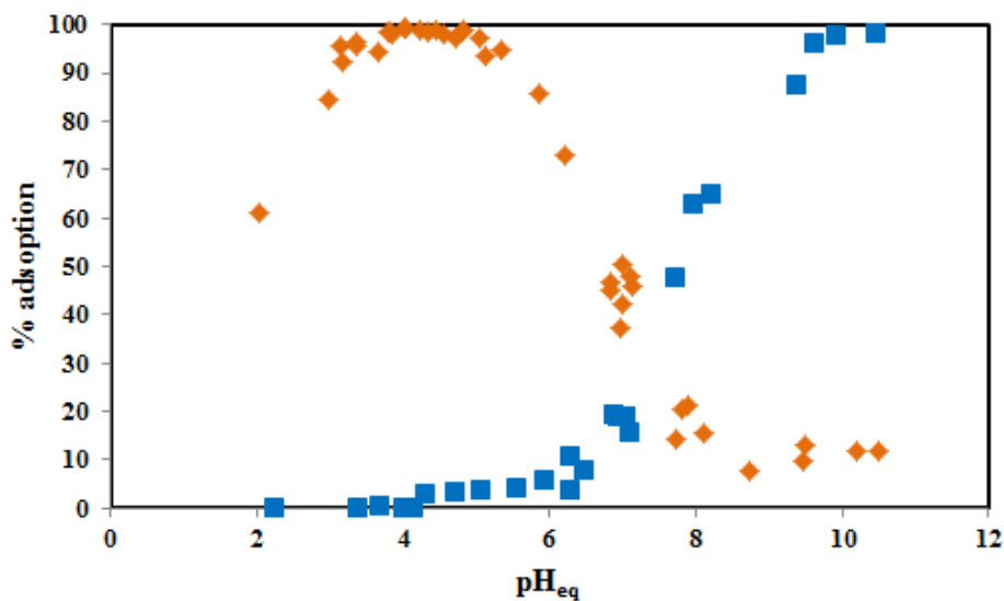
Figure IV.6: effet du pH sur l'adsorption du méthylorange et du bleu de méthylène par les billes de chitosane ( m_b=2,2\pm 0,1 \text{ g} ; V=20\text{mL} ; t= 2 \text{ jours} ):
