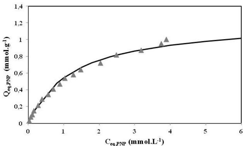
Figure V.18: isotherme d'adsorption du PNP; C_{0,CPC}=1,16\pm 0,01 \text{ mmol.g}^{-1} ( 6,76\pm 0,12 \text{ mmol.L}^{-1} ); m_b \approx 1,075 \text{ g} ; V=10 \text{ mL} ; t=3 \text{ jours} ; Train plein : modélisation par l'équation de Langmuir.
