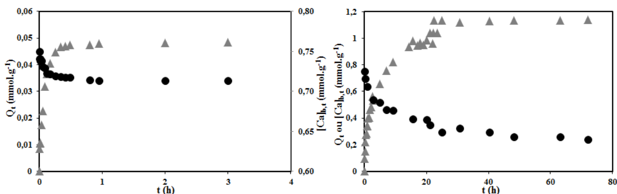
Figure V.11 : cinétique d'adsorption du CPC : Q_t (▲) et [Ca]_{b,t} (●) ; m_b \approx 1,075 \text{ g} ; V=10 \text{ mL} ; pH \approx 7,5 ; Figure de gauche: C_0=0,0492 \pm 0,0002 \text{ mmol.g}^{-1} ( 102,5 \text{ mg.L}^{-1} , 0,286 \text{ mmol.L}^{-1} ) ; Figure de droite: C_0=1,15 \pm 0,01 \text{ mmol.g}^{-1} ( 2,422 \pm 0,006 \text{ g.L}^{-1} ; 6,76 \pm 0,02 \text{ mmol.L}^{-1} ).
