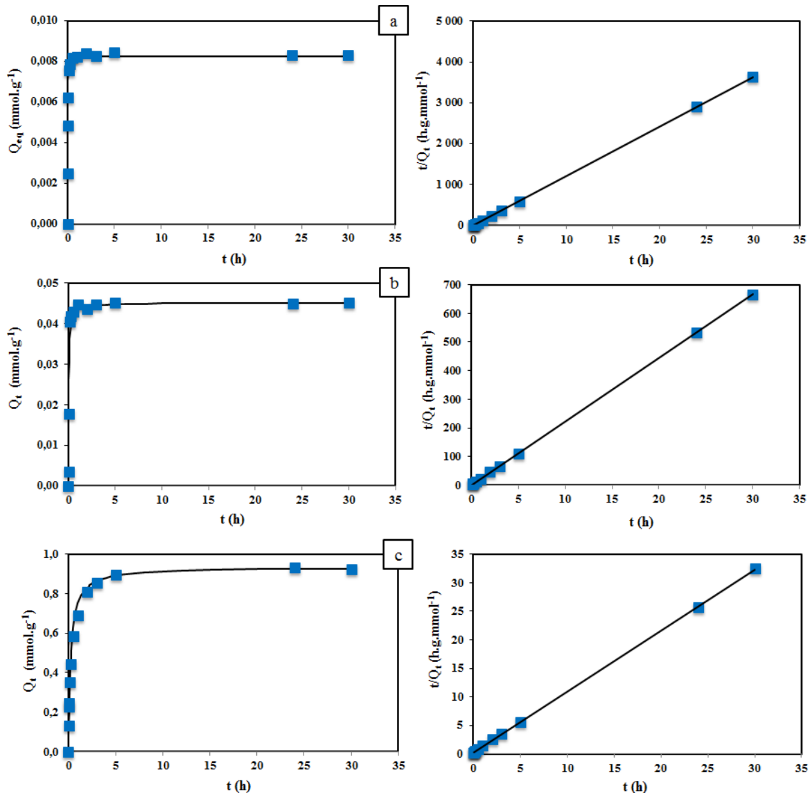
Figure IV.12: cinétique d'adsorption du BM par les billes d'alginate ; m_b \sim 2,15 g ; V=20 mL ; (a) : C_0 = 5,36.10^{-2} mmol.L -1 (0,0095 mmol.g -1 , 20 mg.L -1 ) ; pH=7,0±0,5 (b) : C_0 = 0,267 mmol.L -1 (0,048 mmol.g -1 , 99,8 mg.L -1 ) ; pH=6,6±0,3 (c) : C_0 = 6 mmol.L -1 (1,072 mmol.g -1 , 2,243 g.L -1 ) ; pH=5,6±0,6 ; Trait plein : modélisation par l'équation pseudo-ordre 2.
