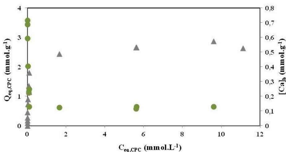
Figure V.17: isotherme d'adsorption du CPC en présence du PNP ( \blacktriangle , axe de gauche) et quantité de calcium dans les billes ( \bullet , axe de droite) ; C_{0,PNP}=103 \text{ mg.L}^{-1} ; t=3 \text{ jours} ; pH_{eq}=6,6\pm 0,3 ; m_b\approx 2,15 \text{ g} ; V=20 \text{ mL} .
