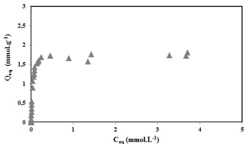
Figure V.6: isotherme d'adsorption du CPC par les billes d'alginate magnétiques; m_b \approx 2,15 \text{ g} ; V=20 \text{ mL} ; pH_{eq}=7,0 \pm 0,5 ; t=3 \text{ jours} .
