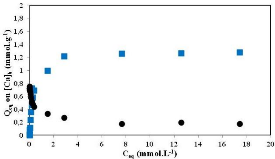
Figure V.10: isotherme d'adsorption du BM par les billes d'alginate magnétiques; Q_{eq} (■); [Ca]_b (●); m_b=2,149\pm 0,004 \text{ g} ; t=2 \text{ jours} ; pH_{eq}=6,8\pm 0,2 ; V=20 \text{ mL} .
