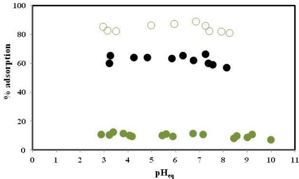
Figure VI.6: Effet du pH sur l'adsorption du PNP par les billes magnétiques d'alginate : R=0 (●), R=2 (●), R=4 (○); C_0=100 \text{ mg.L}^{-1} ( 0,7 \text{ mmol.L}^{-1} ; 6,76 \cdot 10^{-3} \text{ mmol.g}^{-1} ), m_b=0,530 \pm 0,001 \text{ g} ; V=5 \text{ mL} ; t=2\text{-}3 \text{ jours} .
