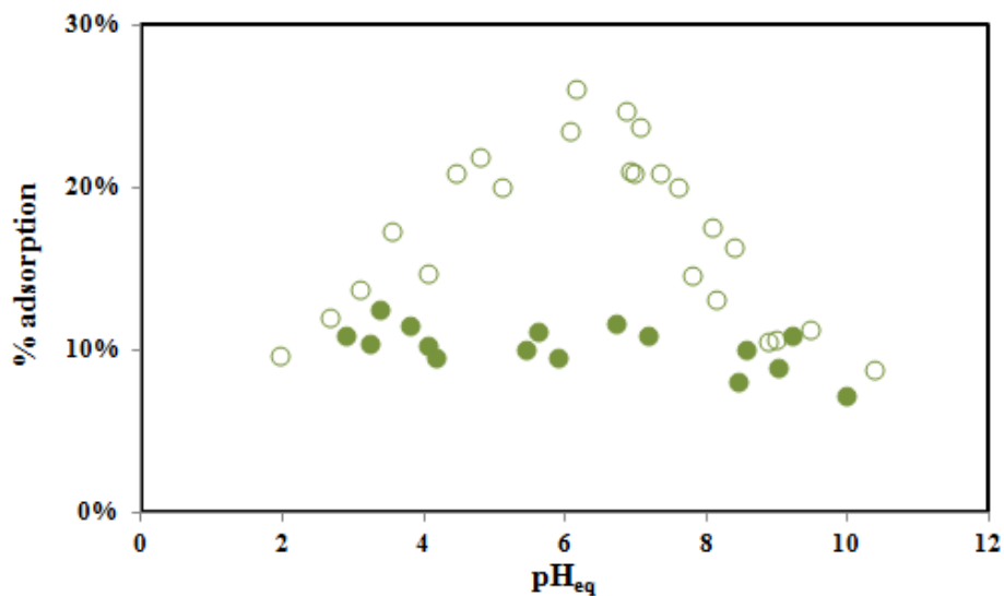
Figure V.1: effet du pH sur l'adsorption du PNP par des billes de chitosane (○) ou d'alginate (●). C_0=0,71\pm 0,07 \text{ mmol. L}^{-1} ( 0,1225\pm 0,0002 \text{ mmol.g}^{-1} ; 99\pm 1 \text{ mg.L}^{-1} ); m_b=2,154\pm 0,004 \text{ g} ; V=20 \text{ mL} ; t=24 \text{ h} .
