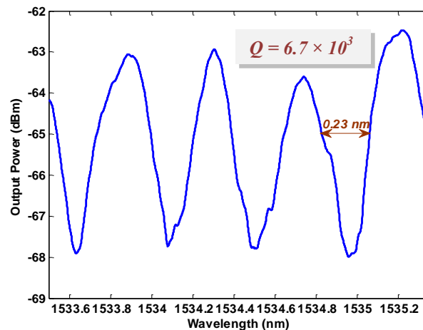
Fig. I.12 Spectre de puissance de sortie pour une gouttelette de diamètre 1,16 mm excitée par un faisceau gaussien avec une taille de rayon de 9 \mu\text{m} . La largeur de bande à 3dB est de 0,23 nm, le facteur de qualité total est de 6,7 \times 10^3 .
