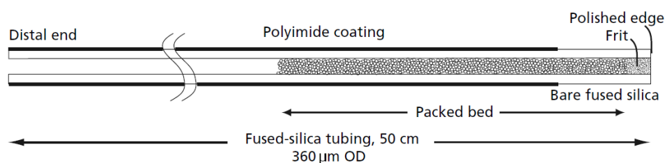
Fig. 6.1 IntegraFrit™ Column [5].
