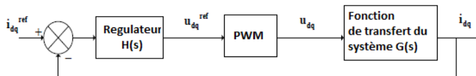
FIGURE D.4 – Boucle de commande des courants
