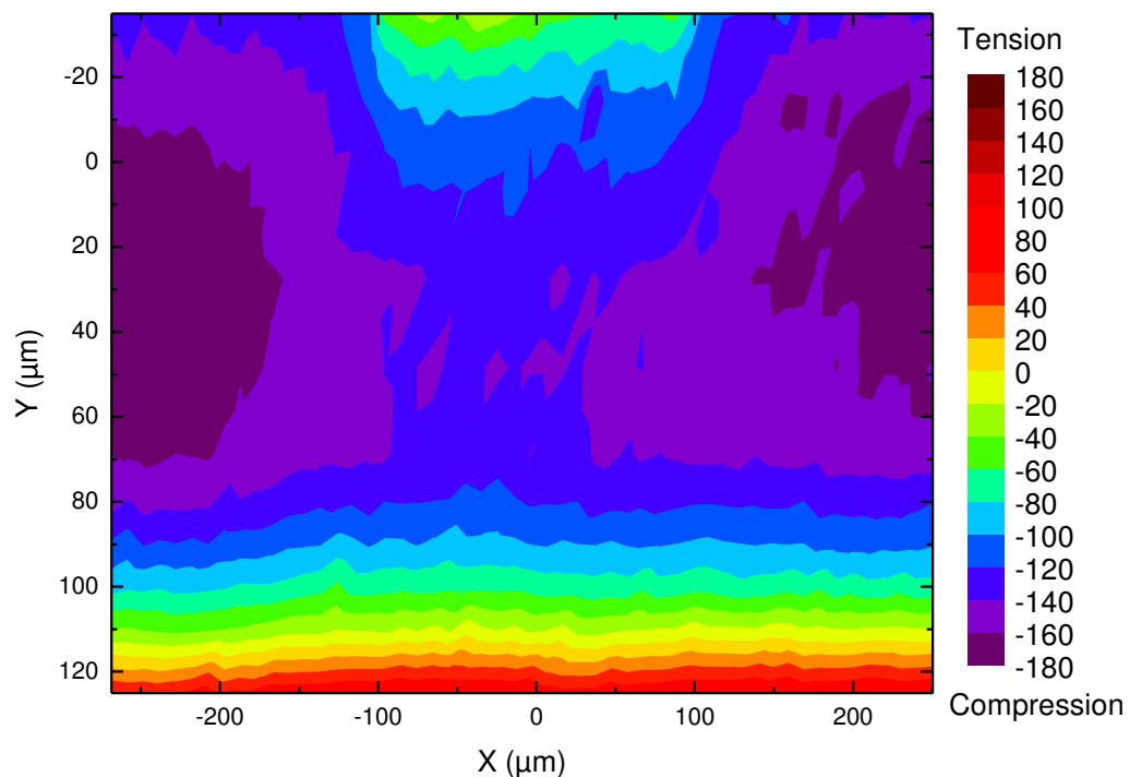
Fig II.10 Champ de contrainte de la diode de puissance en MPa
