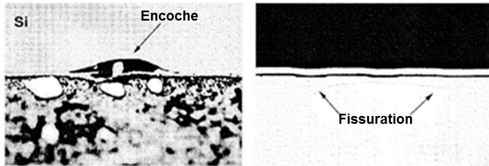
Fig I. 8 Encoche dans la puce de silicium (à gauche) ; Fissuration dans la puce de silicium causée par le stress de flexion (micro-section optique image300x) (à droite) [Cia00]
