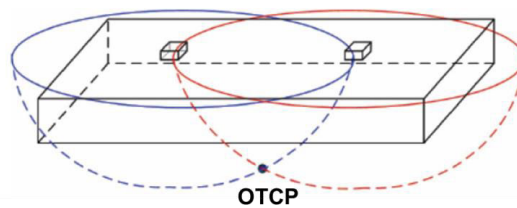
Fig I.38 Prise en compte du couplage thermique entre deux sources de chaleur [Hab05c]
