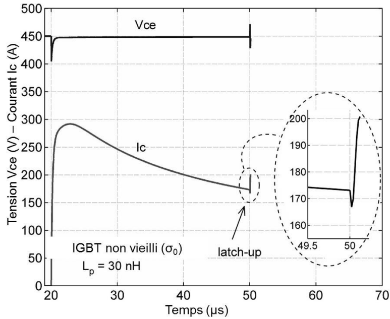
Fig IV.21 Destruction de l'IGBT non vieilli ( L_p = 30\text{nH} )
