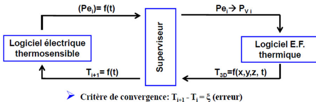
Fig I.27 Schéma de principe de la modélisation électrothermique couplée [Sau09]
