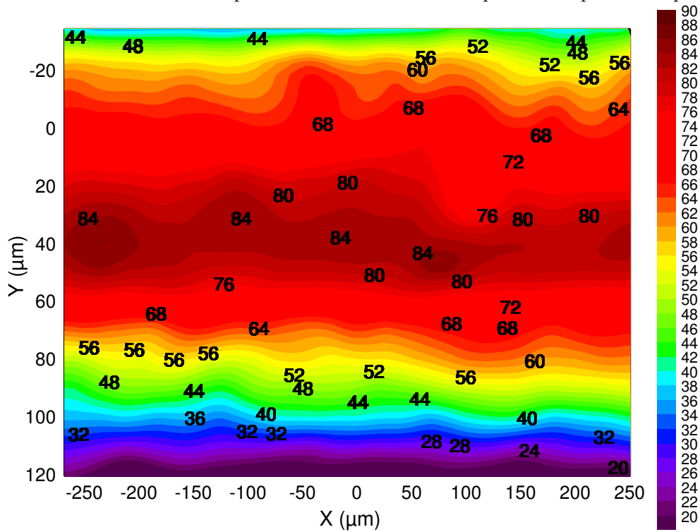
Fig II.18 Répartition de la température dans une micro-section de diode polarisée à 2.83 V / 6 A
