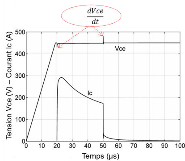
Fig IV.14 Formes d'ondes de court-circuit de l'IGBT NPT (SGP30N60 30A / 600 V)
