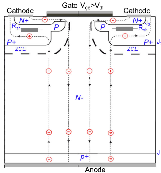
Fig I.10 Trajectoires des porteurs des charges dans une structure IGBT en polarisation directe
