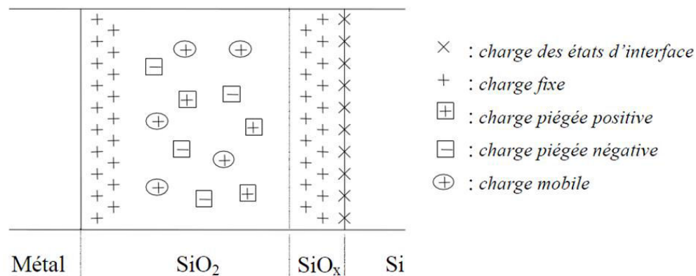
Fig I.12 Les types de charges de l'oxyde et leur site [Man92]
