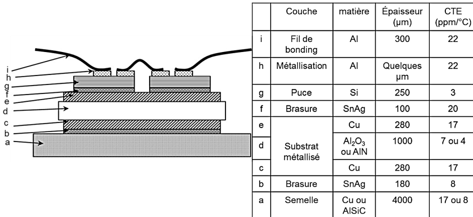
Fig III.1 Structure et matériaux utilisés dans les modules IGBT [Cia02]
