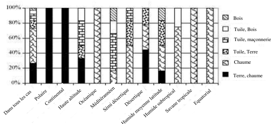
FIGURE 1.1 – Typologie de toiture selon la zone climatique, ( Zhai and Previtali, 2010 )
