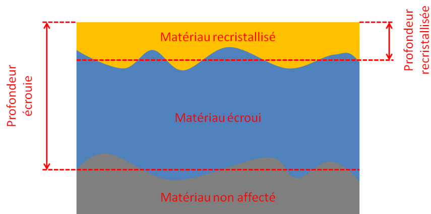
Figure III-28. Représentation schématique des modifications microstructurales de la subsurface sous la trace d'usure. Vue en coupe, la surface est au dessus.
