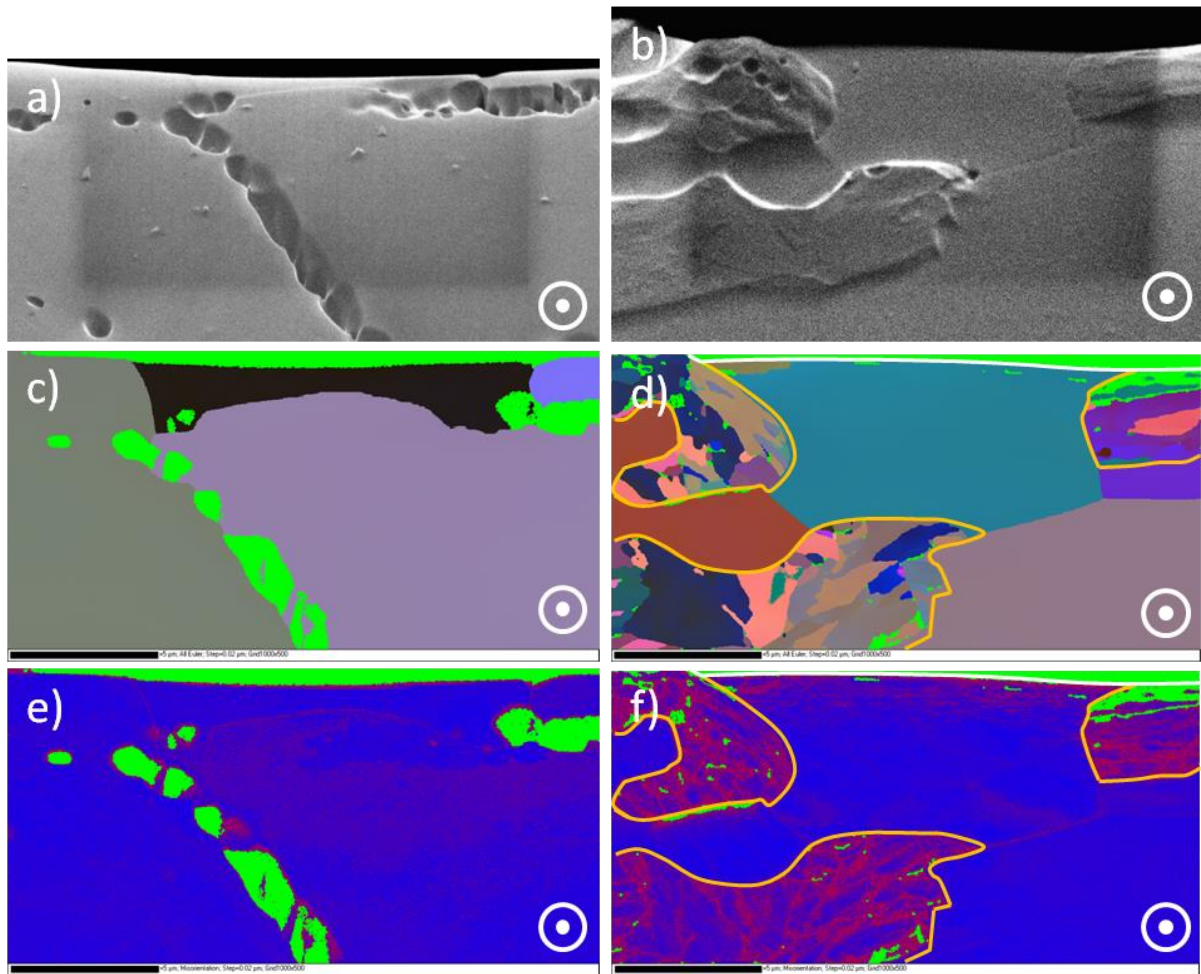
Figure E-9. Analyses EBSD pour les expériences réalisées à -0,710 V/MSE : images post acquisitions pour a) le ferritique (F) et b) le ferrito-martensitique (FM), cartes d'orientations en représentation d'Euler pour c) le F et d) le FM, cartes de désorientation locale pour e) le F et f) le FM. La barre d'échelle représente 5 \mu\text{m} . La direction de frottement est indiquée par les flèches. Les échantillons étant électropolis, les carbures sont déchaussés de la matrice ferritique.
