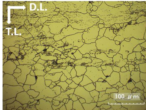
Figure I-3. Microstructure de l'acier inoxydable ferritique, révélée après attaque électrochimique. Les directions de laminage (D.L.) et transverse au laminage (T.L.) sont indiquées par les flèches blanches.
