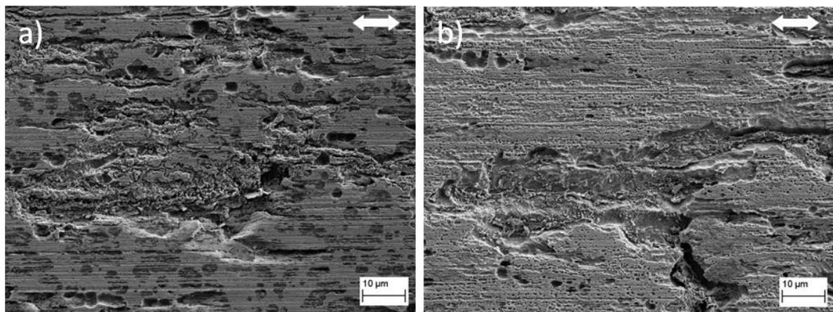
Figure III-18. Observations MEB du milieu de la trace d'usure après des essais effectués à -0,950 V/MSE pour a) le ferritique (F) et b) le ferrito-martensitique (FM). Les flèches indiquent la direction du frottement.
