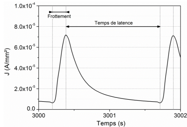
Figure II-21. Evolution de la densité de courant au cours du temps, enregistré pour un échantillon ferritique en milieu acide avec un temps de latence de 1,2 s.
