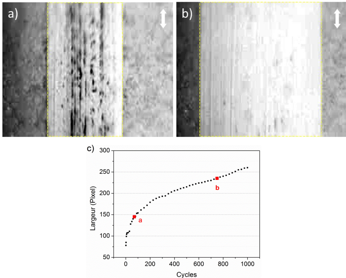
Figure II-8. Suivi optique de la trace d'usure a) pendant la période de rodage et b) une fois le régime stationnaire de l'usure atteint. Les zone définies par les pointillés jaune indiquent les largeurs extraites à partir des images ; c) évolution de la largeur de la trace d'usure en fonction du nombre de cycles, les mesures correspondant aux images a) et b) sont indiquées en rouge.
