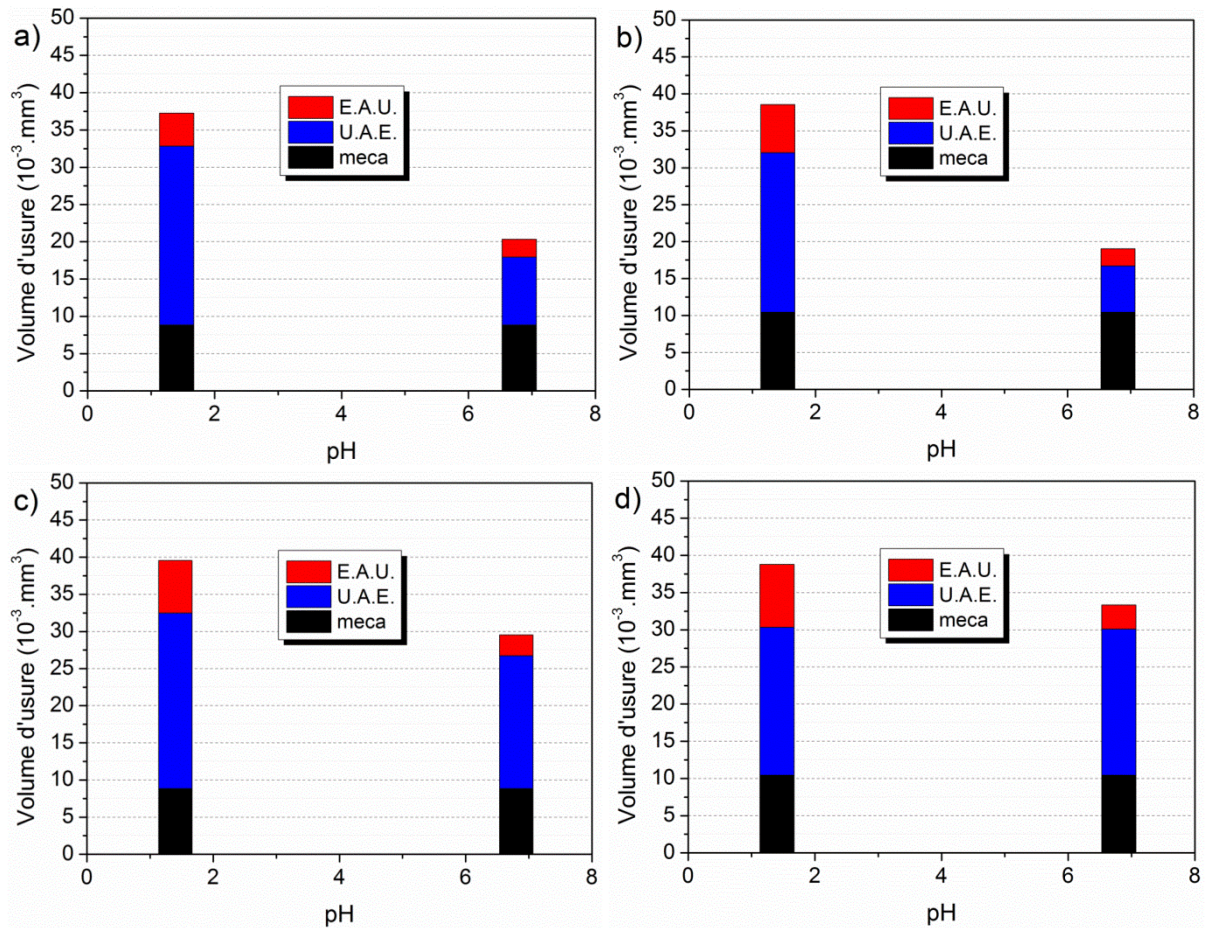
Figure III-47. Détail des volumes d'usure avec un temps de latence de 1,2 s pour l'acier inoxydable a) ferritique (F) et b) ferrito-martensitique (FM) ; avec un temps de latence de 5,7 s pour c) le F et d) le FM.
