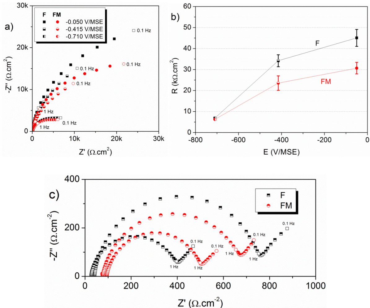
Figure III-10. Mesures de spectroscopie d'impédance électrochimique pour les aciers inoxydables ferritique (F) et ferrite-martensitique (FM) tracées dans des diagrammes de Nyquist pour a) les potentiels du plateau passif avec b) les résistances interfaciales spécifiques associées et c) pour le potentiel du domaine de dissolution anodique.
