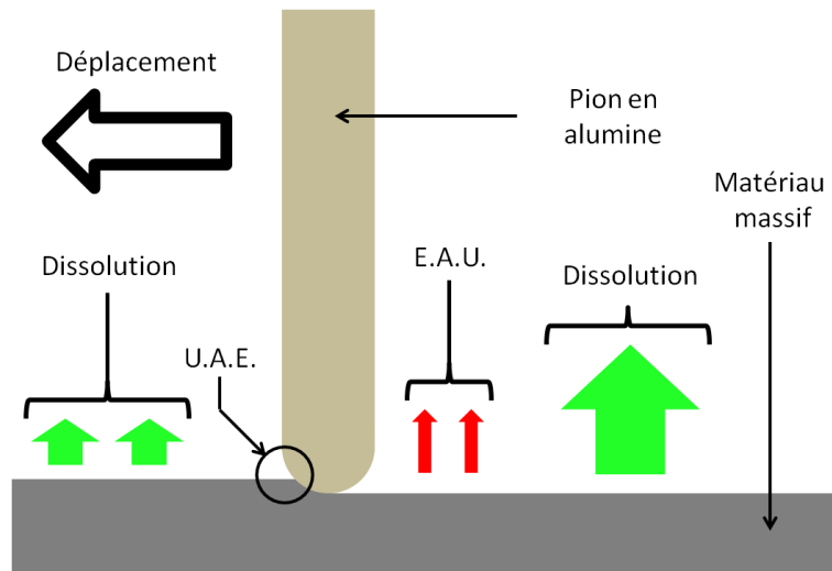
Figure I-28. Représentation schématique de l'usure de la surface de l'échantillon par le déplacement du pion sous potentiel imposé dans le domaine de dissolution anodique.
