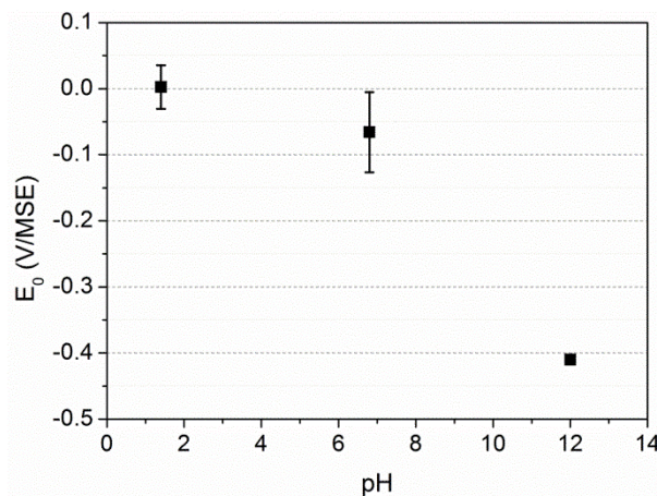
Figure II-13. Potentiel avant frottement ( E_0 ) pour les essais effectués en potentiel libre.
