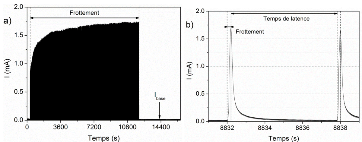
Figure I-20. Evolution du courant en fonction du temps lors d'un essai effectué sous polarisation anodique à -0,050 \text{ V/MSE} a) sur la totalité de l'expérience et b) sur une durée réduite.
