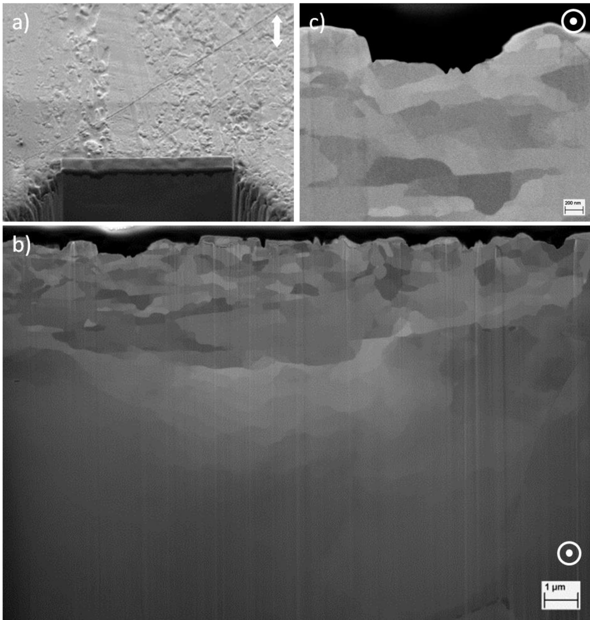
Figure E-13. Découpe FIB de l'échantillon F à -0,710 \text{ V/MSE} a) localisation de la position de la coupe dans la trace avec le détecteur SE b) vue générale de la coupe avec le détecteur SE c) détail sur la gauche de la coupe avec le détecteur BSE. La direction de frottement est indiquée par les flèches.
