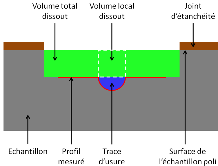
Figure I-27. Représentation schématique de l'usure de la surface de l'échantillon sous potentiel imposé dans le domaine de dissolution anodique.
