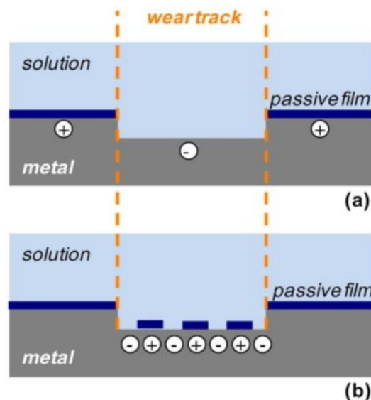
Figure II-5. Représentation schématique de situations de couplage galvanique pouvant se produire en tribocorrosion en potentiel libre a) entre une trace d'usure complètement dépassivée et l'aire environnante et b) entre des zones dépassivées et d'autres encore passives au sein de la trace d'usure.
