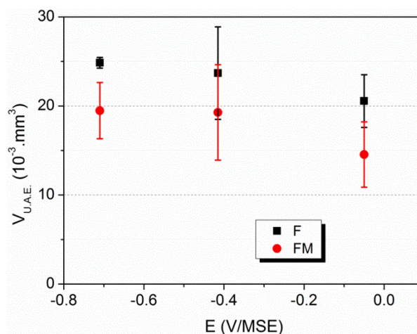
Figure III-21. Evolution du volume d'usure accéléré par l'électrochimie ( V_{U.A.E.} ) en fonction du potentiel appliqué dans le domaine passif de comportement des aciers inoxydables ferritique (F) et ferrito-martensitique (FM).
