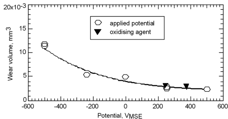
Figure I-1. Volumes d'usure d'un acier inoxydable ferritique dans H_2SO_4 0,5 M [2]. ○ représentent les volumes d'usure obtenus sous différents potentiels imposés VMSE en mV/MSE. ▼ représentent les volumes d'usure obtenus en potentiel libre avec l'ajout de Ce^{4+} à 0,005 et 0,05 M correspondant à des potentiels respectifs de 240 et 380 mV/MSE.
