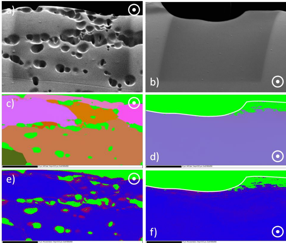
Figure III-33. Analyses EBSD pour les expériences réalisées à -0,865 V/MSE : images post acquisitions pour a) le ferritique (F) et b) le ferrito-martensitique (FM), cartes d'orientations en représentation d'Euler pour c) le F et d) le FM et cartes de désorientation locale pour e) le F et f) le FM. La ligne blanche représente la surface. La barre d'échelle représente 5 \mu\text{m} . La direction de frottement est indiquée par les flèches. Les échantillons étant électropolis, les carbures sont déchaussés de la matrice ferritique.
