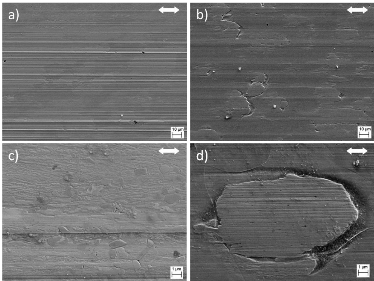
Figure E-3. Observations MEB du milieu de la trace d'usure après des essais effectués à -0,710 V/MSE pour a) le ferritique (F) et b) le ferrito-martensitique (FM) ; détail de la surface pour c) le F et d) le FM. Les flèches indiquent la direction du frottement.
