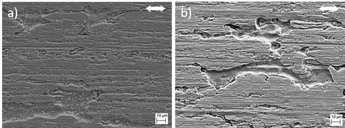
Figure E-2. Observations MEB après des essais effectués à -0,865 V/MSE au milieu de la trace d'usure pour a) le ferritique et b) le ferrito-martensitique. Les flèches indiquent la direction du frottement.
