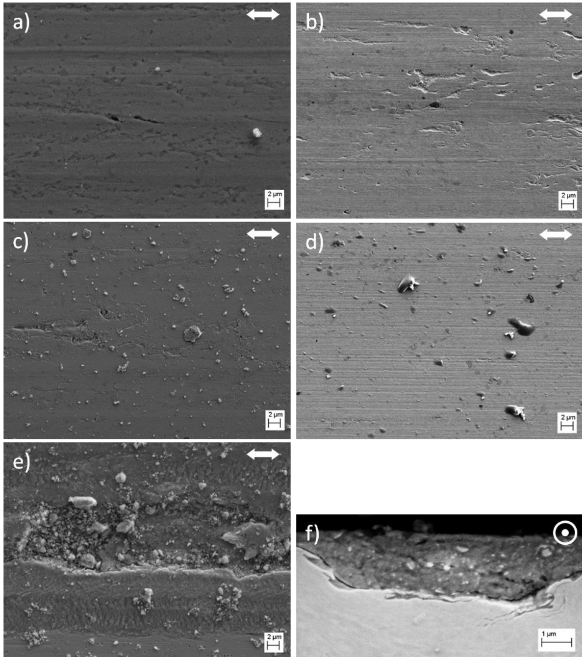
Figure II-18. Observations MEB de la trace d'usure pour des expériences réalisées en milieu acide avec un temps de latence de a) 5,7 et b) 1,2 s ; en milieu neutre avec un temps de latence de c) 5,7 et d) 1,2 s ; en milieu basique avec un temps de latence de 5,7 s e) vue de dessus et f) vue en coupe.
