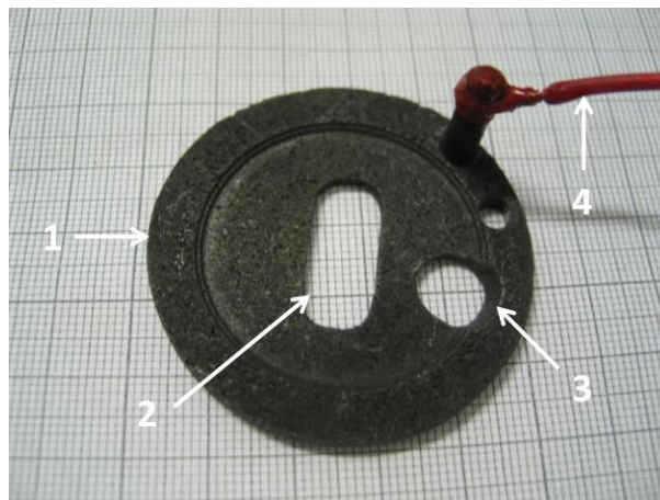
Figure I-10. Contre électrode en graphite. 1) Contre électrode 2) Ouverture permettant le mouvement du pion 3) Ouverture permettant le placement de l'électrode de référence 4) Contact électrique.
