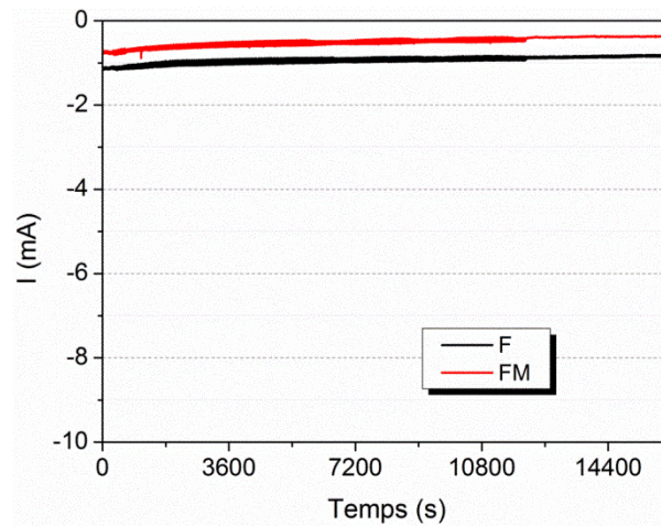
Figure III-17. Evolution du courant lors des essais de tribocorrosion -0,950 V/MSE sur les aciers inoxydables ferritique (F) et ferrito-martensitique (FM).
