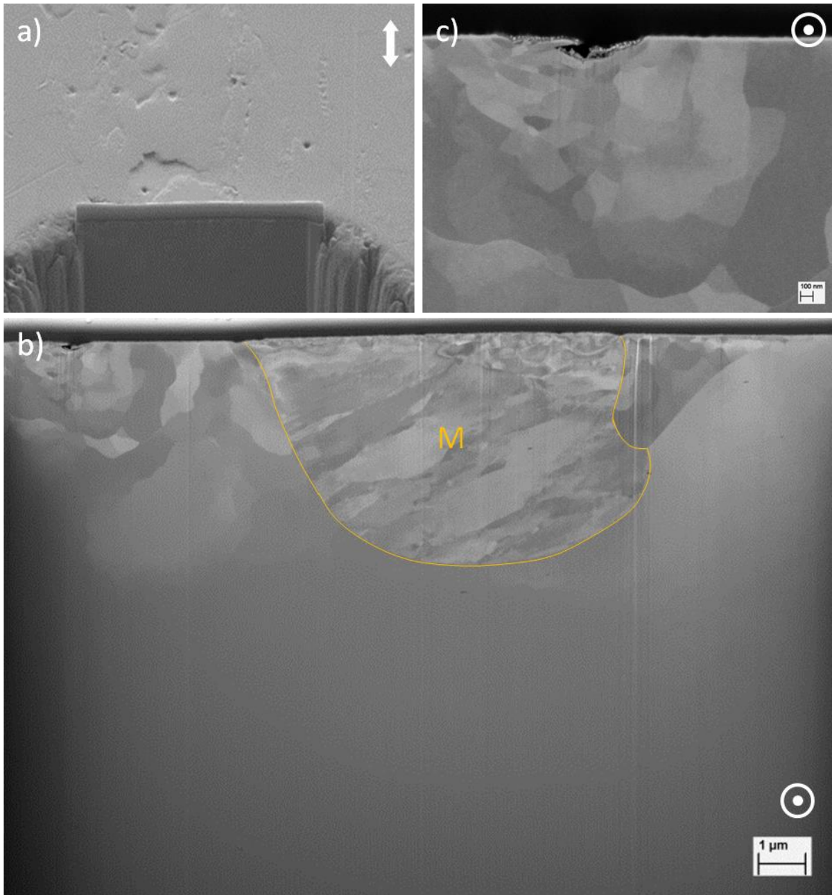
Figure E-14. Découpe FIB de l'échantillon FM à -0,710 \text{ V/MSE} a) localisation de la position de la coupe dans la trace avec le détecteur SE b) vue générale de la coupe avec le détecteur SE c) détail sur la gauche de la coupe avec le détecteur BSE. La direction de frottement est indiquée par les flèches.
