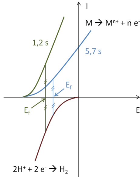
Figure II-16. Représentation schématique de l'évolution du potentiel de corrosion E_f suivant le temps de latence en milieu acide.
