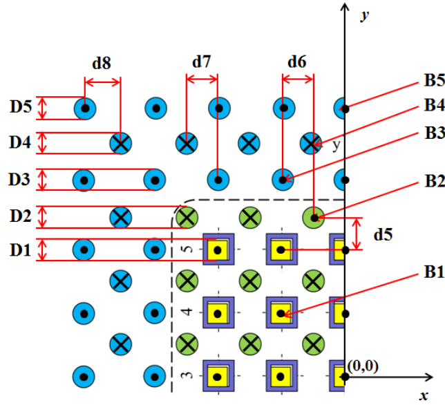
Fig IV-4: 14 design parameters
