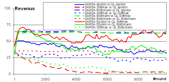
(d) Revenus en utilisant le SARSA contre un adversaire qui utilise le Q-Learning
