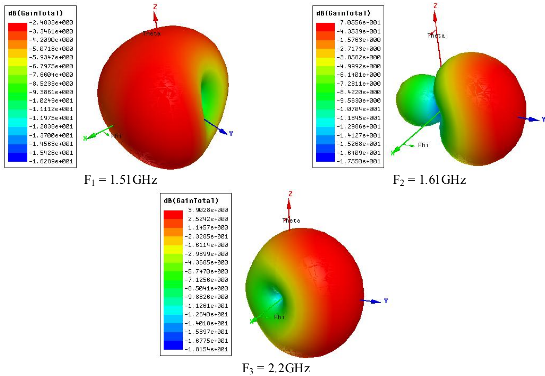
Antenne A2
