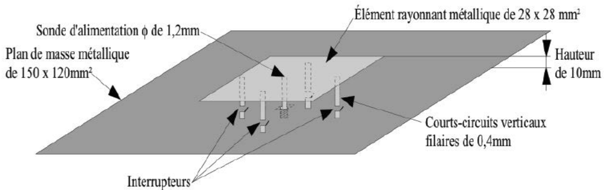
Figure I.23: Exemple d'antenne patch à courts-circuits commutables.
