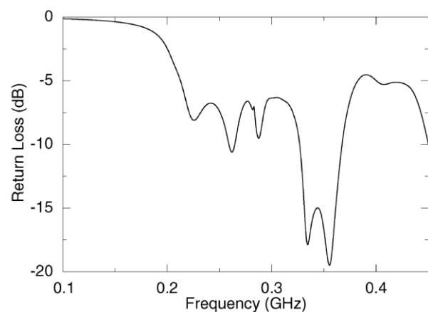
Figure I.8: Exemple d'antenne à matériaux magnéto-diélectriques : (a) Antenne réalisée et (b) Coefficient de réflexion.
