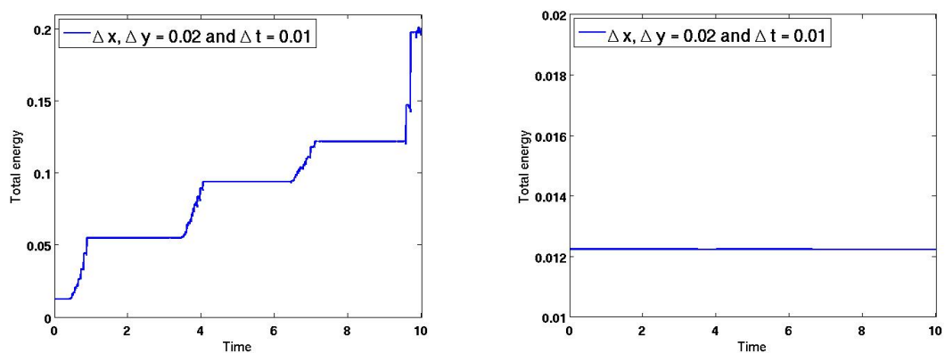
Figure 12: Énergie associée à la solution approchée pour les matrices de masse standard (gauche) et modifiées (droite) avec le schéma de Crank–Nicolson.
