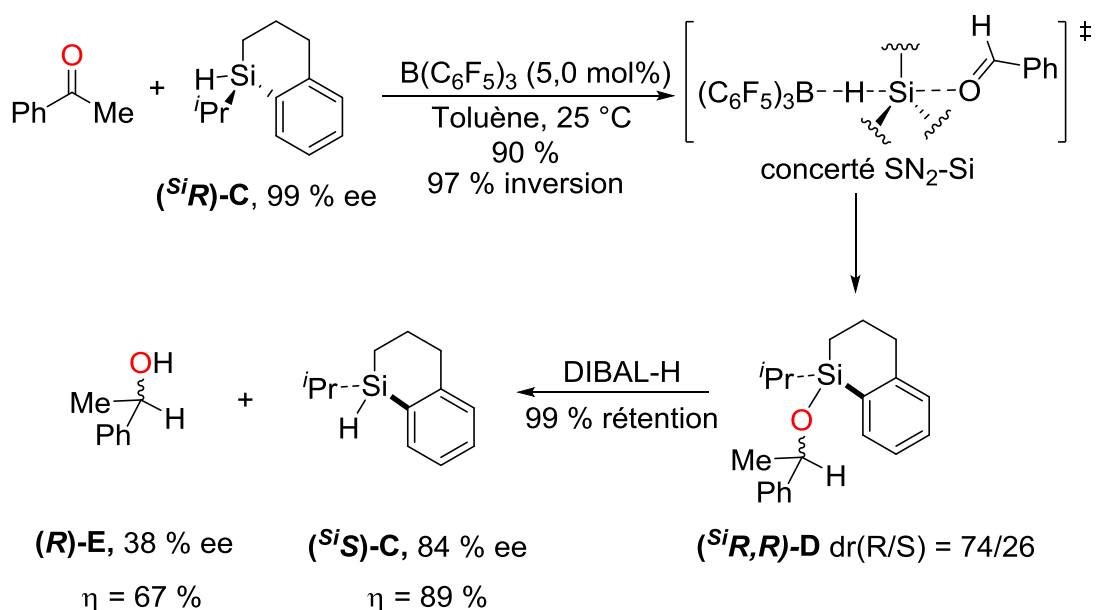
Schéma 3. Hydrosilylation de l'acétophénone catalysée par \text{B}(\text{C}_6\text{F}_5)_3 et avec un hydrosilane contenant un centre stéréogénique. 15
