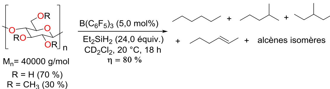
Sch\u00e9ma 7. R\u00e9action de d\u00e9polym\u00e9risation suivie par la d\u00e9soxyg\u00e9nation compl\u00e8te de la cellulose m\u00e9thyl\u00e9e \u00e0 30 % avec le syst\u00e8me \text{B}(\text{C}_6\text{F}_5)_3\text{-Et}_2\text{SiH}_2 .
