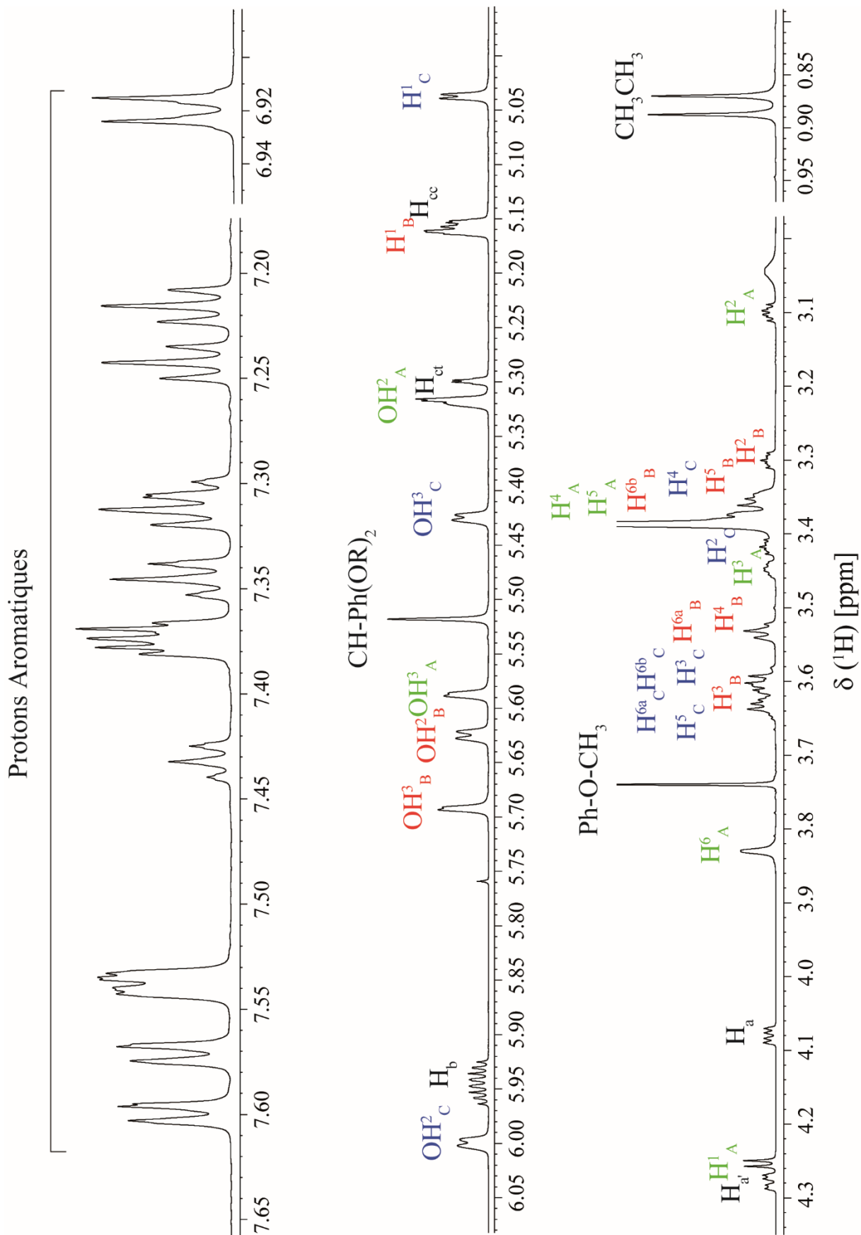
S 2. Le spectre 1 H enregistré à 23,5 T et attribution des protons.
