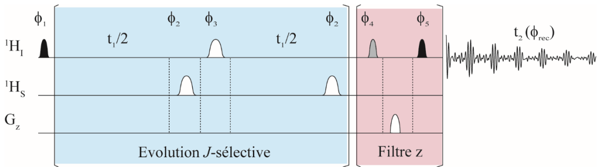
Figure 5. Séquence d'impulsions de l'expérience SERFph. Les formes sinusoïdales noires, grises et blanches sur les canaux ^1\text{H} représentent, respectivement, une impulsion sélective d'excitation, une impulsion sélective « flip-back » et une impulsion sélective de refocalisation. La forme sinusoïdale blanche sur le canal de gradient de champ pulsé G_z , correspond à une impulsion de gradient de forme sinusoïdale. \phi_1 = x, -x ; \phi_2 = x, x, -x, -x ; \phi_3 = x, x, -x, -x ; \phi_4 = -x, x, x, -x ; \phi_5 = x, y, -x, -y ; \phi_{\text{rec}} = y, -x .
