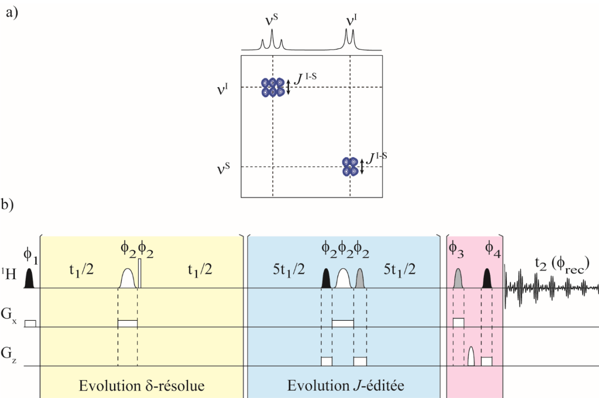
Figure 16. L'expérience PCR-COSY. a) Le spectre théorique de l'expérience PCR-COSY. Seuls les signaux de deux des protons apparaissent sur ce spectre théorique. (b) La séquence d'impulsions de l'expérience PCR-COSY. Sur le canal proton ( ^1\text{H} ), les formes sinusoïdales noires, grises et blanches correspondent respectivement à une impulsion sélective d'excitation \pi/2 , à une impulsion sélective de basculement-retour (« flip-back ») \pi/2 et à une impulsion sélective de refocalisation \pi ; le rectangle blanc correspond à une impulsion non-sélective de refocalisation \pi . Sur les canaux des gradients de champ pulsé ( G_x et G_z ), les rectangles blancs correspondent à l'application d'un gradient de forme rectangulaire (sur x ou z , respectivement) et la forme sinusoïdale blanche correspond à un gradient de forme sinusoïdale sur z . Le cyclage de phase est \phi_1 = (x, x, x, x, -x, -x, -x, -x) ; \phi_2 = x ; \phi_3 = (x, -x) ; \phi_4 = (x, x, -x, -x) et \phi_{\text{rec}} = (x, x, x, x, -x, -x, -x, -x) .
