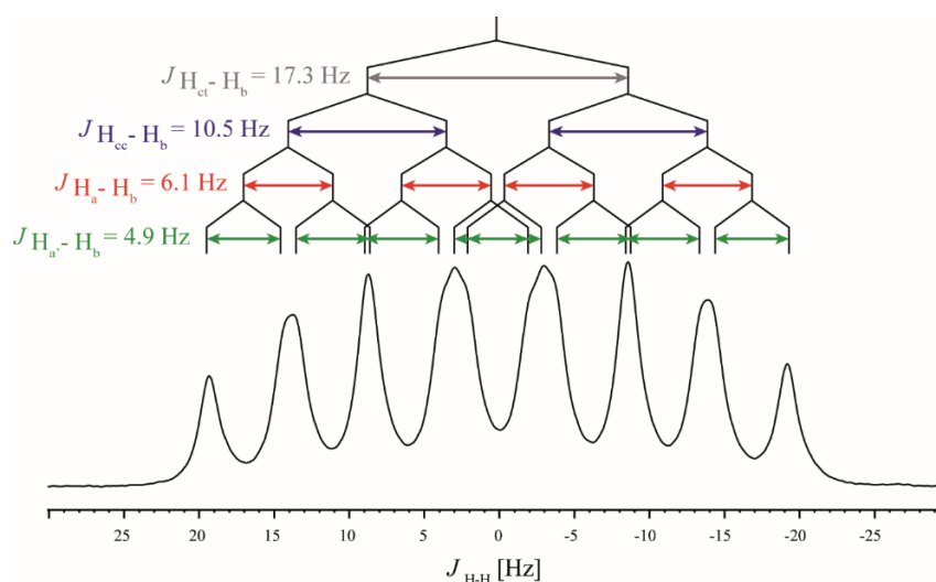
Figure 33. Le détail de la structure fine du multiplet du proton H_b qui peut être déduit des mesures de couplages réalisées sur les données G-SERF ( Figure 32 ). Le signal expérimental correspond au signal du proton H_b observé sur le spectre proton standard enregistré à 23,5 T.
