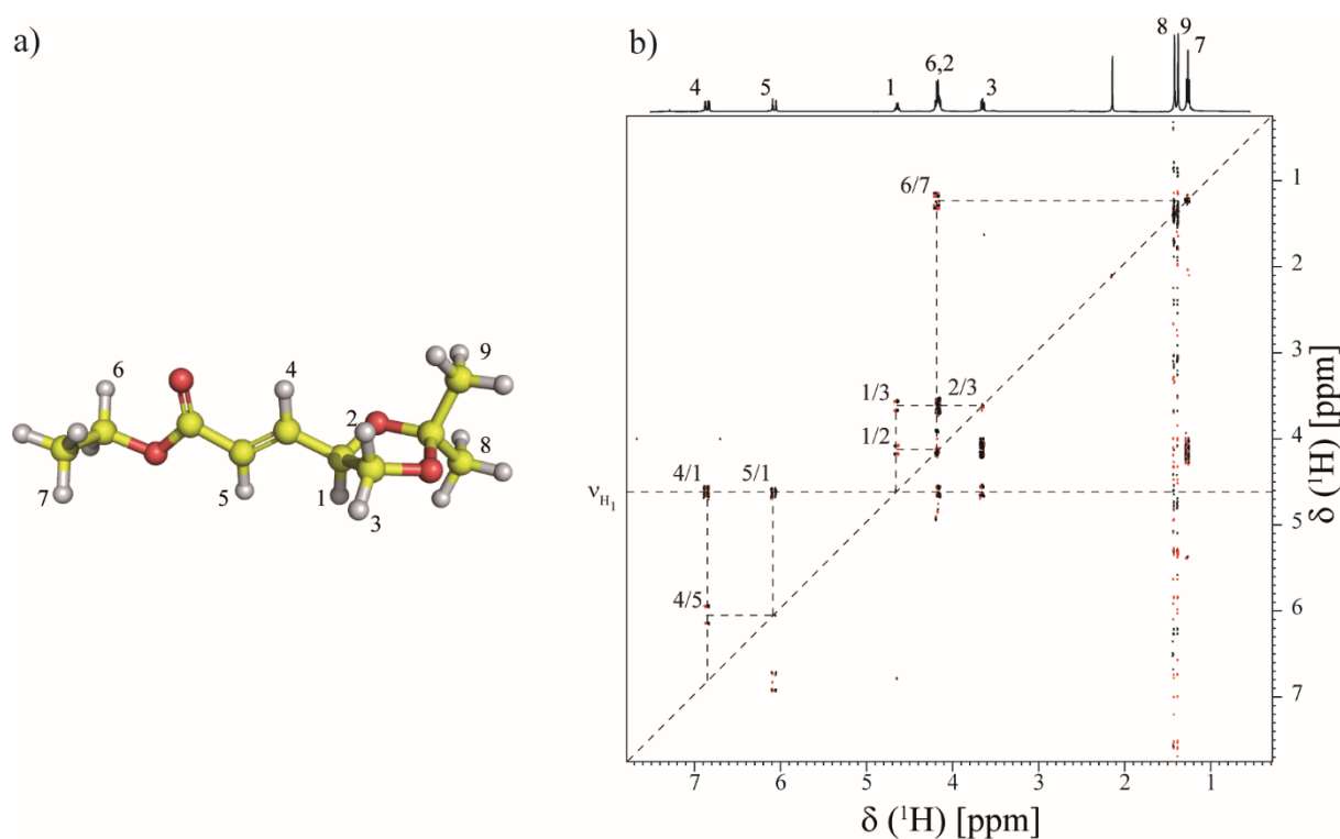
Figure 18. a) Structure de ( \pm )(2,2-diméthyl-1,3-dioxolan-4-yl)3-trans-propenoate d'éthyle. (b) Spectre 2D PCR-COSY enregistré sur cette molécule.
