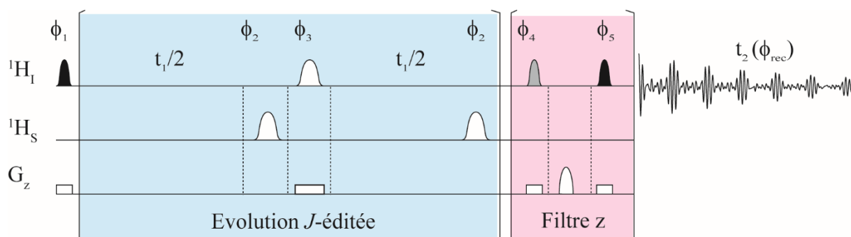
Figure 8. Séquence d'impulsions de l'expérience G-SERFph. Les formes sinusoïdales noires, grises et blanches sur les canaux ^1\text{H} représentent, respectivement, une impulsion d'excitation de 90^\circ , une impulsion flip-back de 90^\circ et une impulsion de refocalisation de 180^\circ . Les rectangles blancs correspondent à un gradient de champ pulsé de forme rectangulaire. La forme sinusoïdale blanche sur le canal G_z correspond à un gradient de champ pulsé de forme sinusoïdale. \phi_1 = x, -x ; \phi_2 = x, x, -x, -x ; \phi_3 = x, x, -x, -x ; \phi_4 = -x, x, x, -x ; \phi_5 = x, y, -x, -y ; \phi_{\text{rec}} = y, -x .
