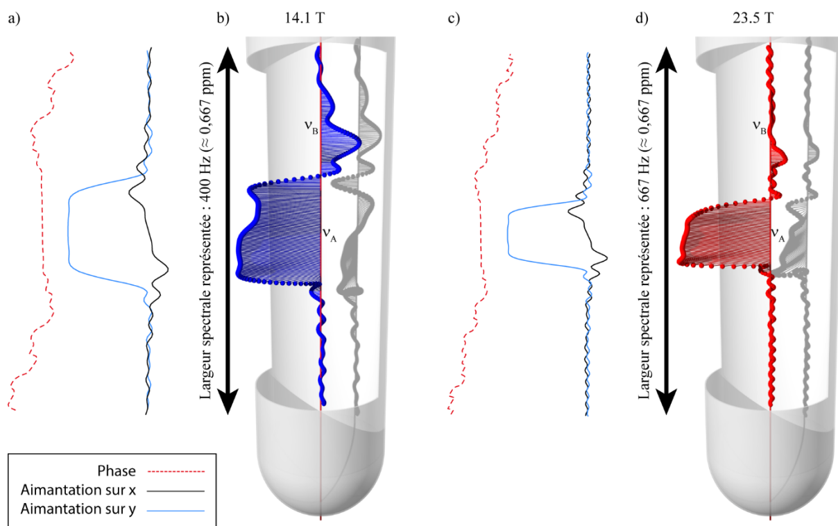
Figure 10. Représentation de l'aimantation d'une unique cohérence du signal du proton H^A . Représentation théorique en 2D de la phase (en rouge) et de l'aimantation selon l'axe x (en noir) et y (en bleu) à (a) 14.1 T et (c) 23,5 T, issu de l'outil « shapetool » de TOPSPIN. Evolution de l'aimantation en 3D calculée dans chaque coupe virtuelle à la fin de l'impulsion d'excitation sélective encodée d'une durée de 50 ms, pour la cohérence A_+B_\alpha X_\alpha du spin du proton H^A à (b) 14,1T et (d) 23,5 T. Une impulsion modulée EBurp2 de 1000 points a été utilisée pour l'excitation sélective. L'échantillon virtuel est divisé en 1521 coupes de taille égale. (Seules les 507 coupes encodées autour des déplacements chimiques de H^A et H^B sont affichées).
