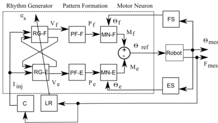
Figure 92. Modèle complet du contrôleur CPG pour une articulation du robot.
