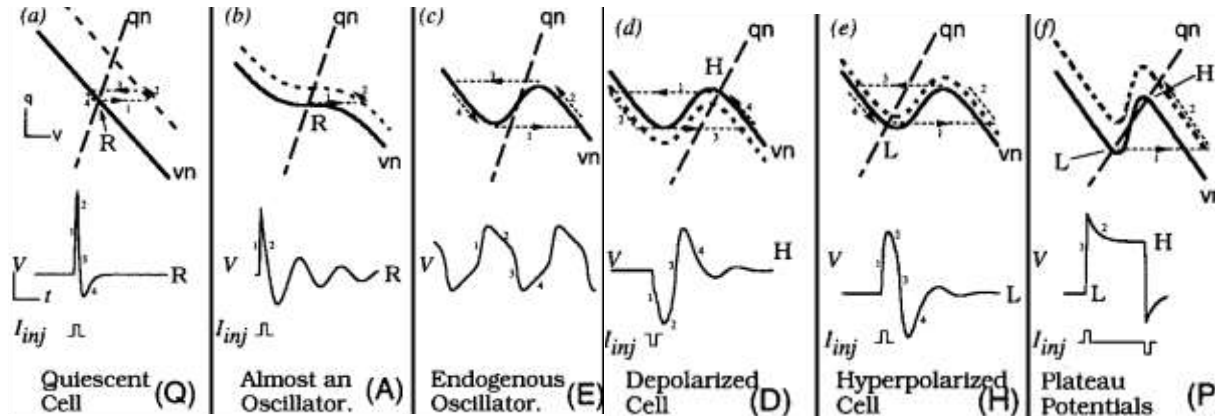
Figure 65. Six comportements intrinsèques du modèle cellulaire de Rowat-Selverston: Q, A, E, D, H, P. Chaque boîte montre le portrait de phase sur le phase plane (V, q), le courbe de potentiel membranaire correspondante à ce plane et le courbe de I inj . Les V et Q nullclines sont étiquetés avec vn (trait plein) et qn (tirets longs). (extrait de (Rowat & Selverston, 1997))
