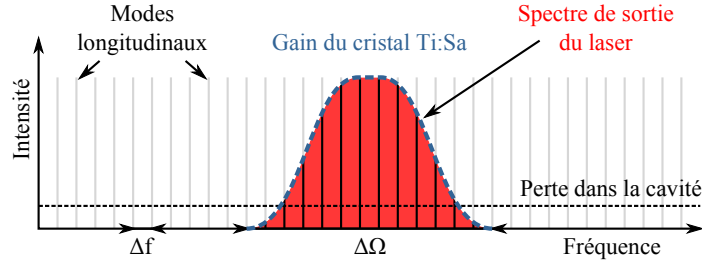
FIGURE 1.1 – Représentation de la bande passante d'un laser femtoseconde en fonction du gain du cristal Ti:Sa et de la cavité de Fabry-Pérot, générant les modes longitudinaux.
