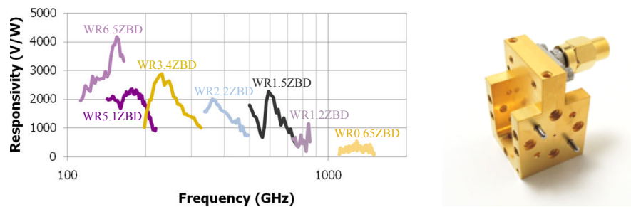
FIGURE 1.32 – Couverture spectrale des diodes Schottky Virginia Diodes, à gauche et photo type d'un dispositif tel qu'il est livré (blindé), à droite.
