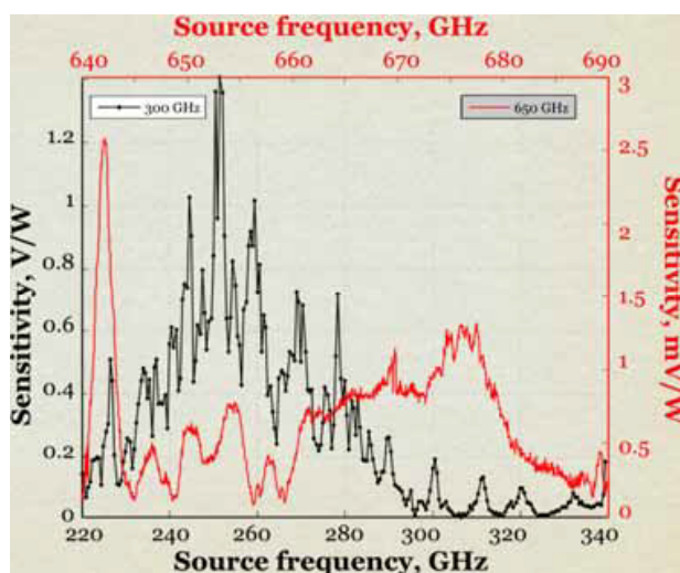
FIGURE A.7 – Résultat de la réponse du transistor HP obtenue à l'aide d'une source électronique continue accordable en fréquence et mesurée avec un analyseur de spectre.
