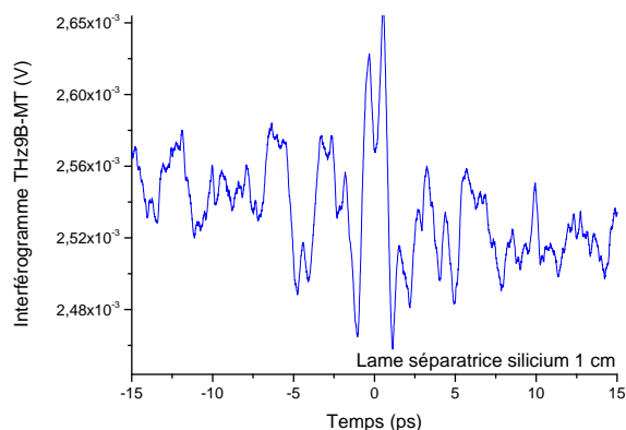
FIGURE 2.31 – Interférogramme mesuré par le pyromètre THz9B-MT avec une séparatrice en silicium d'épaisseur 1 cm et le Tera-Sed 10 en émission.
