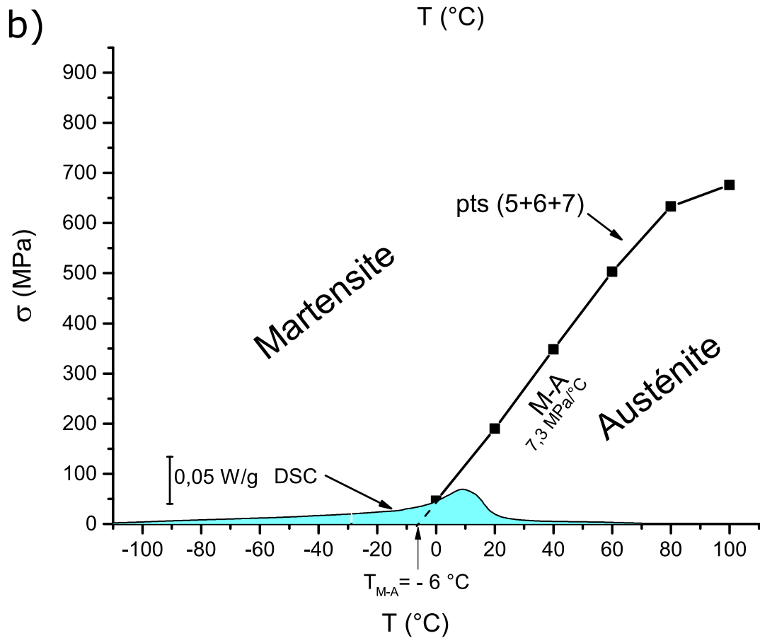
FIGURE 3.42: Tracé des points caractéristiques lors du déchargement a) identification des phases, b) estimation des températures de transformation.
