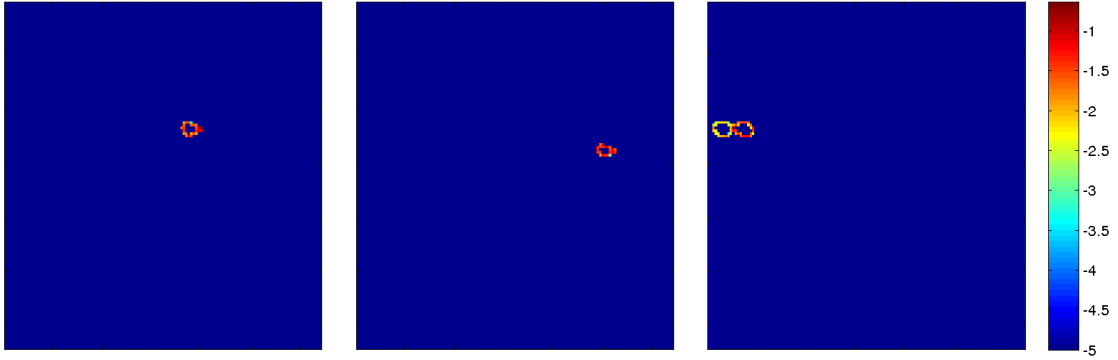
FIGURE 1.3: Densité de la mesure invariante canonique \mu_x^{f_N} de f_N , obtenue comme limite au sens de Cesàro des poussés en avant par f_N de la mesure \delta_x , avec x = (1/2, 1/2) . La densité est représentée en échelle logarithmique : un pixel orange porte une mesure d'environ 10^{-2} . L'homéomorphisme f est une petite perturbation C^1 de l'identité (voir la section 12.3). De gauche à droite, N = 2^{20} + 1, 2^{20} + 2, 2^{20} + 3 .
