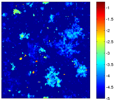
FIGURE 13.3: Densité de la mesure \mu_{\mathbb{T}^2}^{f_N} , pour f un exemple d'homéomorphisme dissipatif proche de l'identité avec de petits ensembles attractifs, et N = 32768 (voir page 66 pour la définition de cet homéomorphisme).
