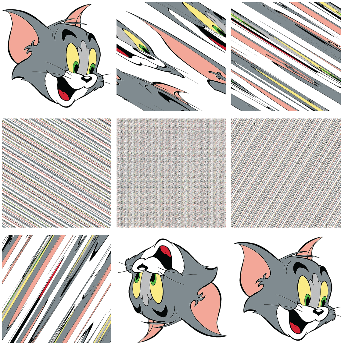
FIGURE 1.1: Images d'une image de chat par la discrétisation du chat d'Arnold, sur une grille de taille 610 \times 610 . De gauche à droite et de bas en haut, temps égaux à 0, 2, 4, 8, 14, 20, 26, 30 et 60.
