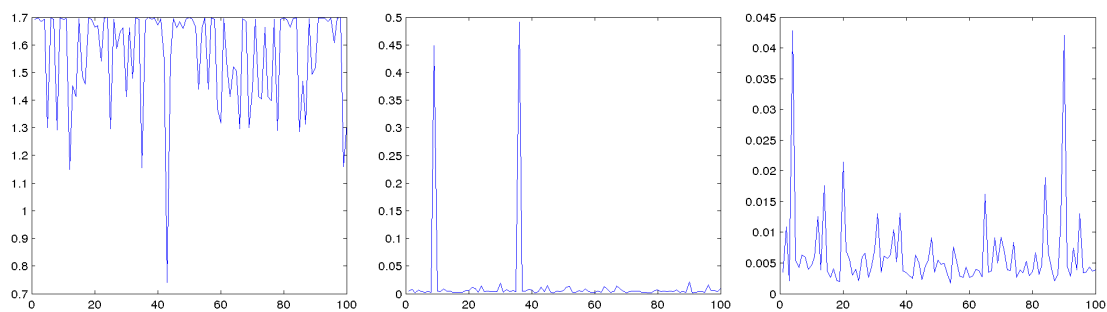
FIGURE 13.5: Distance entre la mesure de Lebesgue et les mesures \mu_x^{(f_i)_N} en fonction de N , for f_1 une petite perturbation de \text{Id} en topologie C^1 (gauche), f_2 une petite perturbation d'une translation d'ordre 30 en topologie C^1 (milieu) et f_3 une petite perturbation d'un automorphisme d'Anosov linéaire en topologie C^1 (droite), sur les grilles E_N , avec N = 2^{20} + k , k = 1, \dots, 100 (voir page 274 pour une définition précise de ces difféomorphismes).
