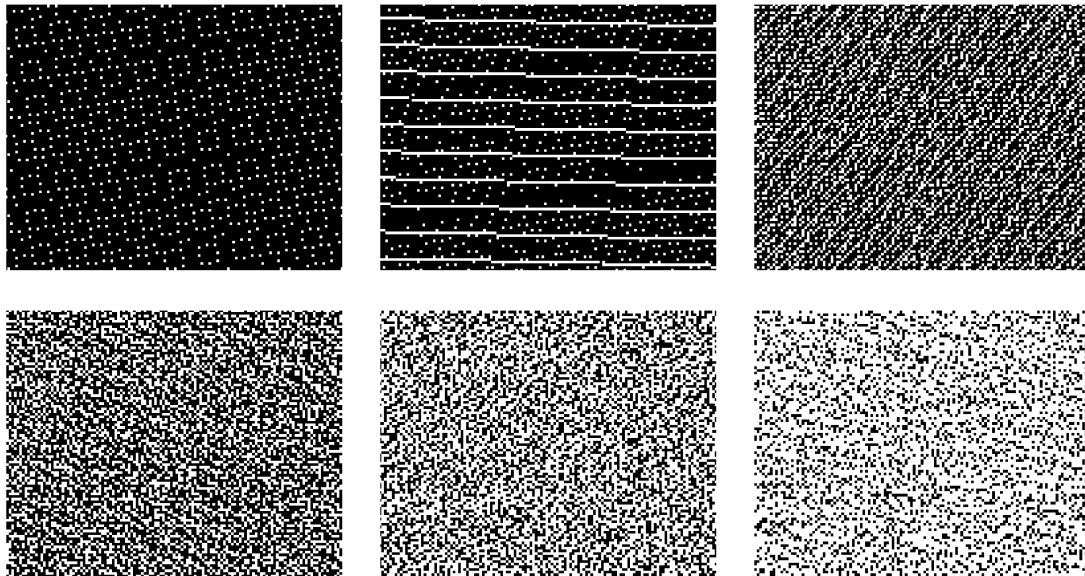
FIGURE 13.1: Images successives de \mathbf{Z}^2 par les discrétisations de k matrices de \mathrm{SL}_2(\mathbf{R}) choisies aléatoirement parmi un compact de \mathrm{SL}_2(\mathbf{R}) (voir la figure 7.2 pour une explication précise). Un point de \mathbf{Z}^2 est noir s'il appartient à l'image. De gauche à droite et de haut en bas, k = 1, 2, 3, 5, 10, 20 .
