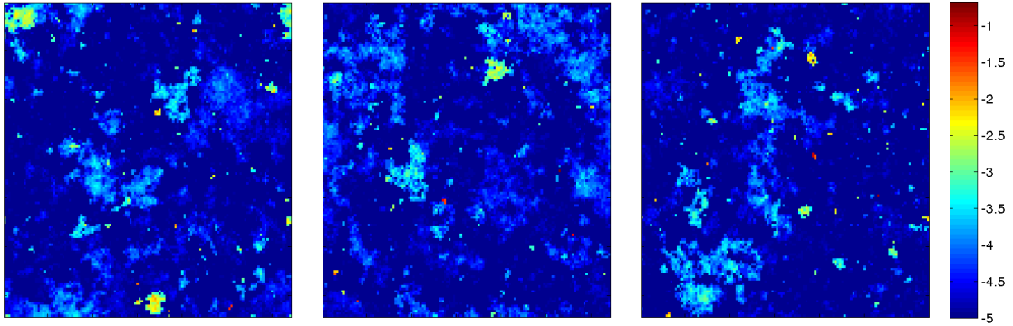
FIGURE 1.2: Densité de la mesure invariante canonique \mu_{\mathbb{T}^2}^{f_N} de f_N , obtenue comme limite au sens de Cesàro des poussés en avant par f_N de la mesure uniforme sur E_N . La densité est représentée en échelle logarithmique : un pixel orange porte une mesure d'environ 10^{-2} . L'homéomorphisme f est une petite perturbation C^0 de l'identité (voir page 99). De gauche à droite, N = 20\,000, 20\,001, 20\,002 .
