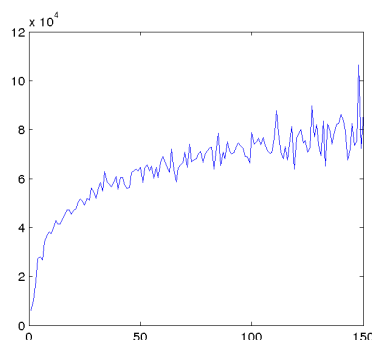
FIGURE 13.2: Cardinal de l'ensemble récurrent \Omega(f_N) en fonction de N , pour N = 128k , k = 1, \dots, 150 , et f un exemple d'homéomorphisme conservatif proche de l'identité (voir page 99 pour la définition de cet homéomorphisme).
