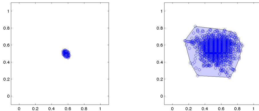
FIGURE 1.4: Comparaison des méthodes de calcul de l'ensemble de rotation sur un même homéomorphisme f « quelconque » (voir sa définition section 6.4). À gauche, ensemble obtenu à l'aide de l'algorithme naturel, qui consiste à calculer des vecteurs de rotation d'orbites très longues. À droite, ensemble obtenu en accumulant les ensembles de rotation de discrétisation sur différentes grilles. Les temps de calcul sont similaires (environ 4h).
