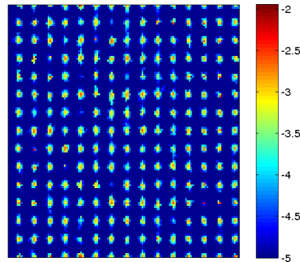
FIGURE 13.4: Densité de la mesure \mu_{\mathbb{T}^2}^{f_N} , pour f un exemple d'homéomorphisme dissipatif proche de l'identité avec de gros ensembles attractifs, et N = 32768 (voir page 66 pour la définition de cet homéomorphisme).
