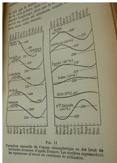
Figure 4 : Variations annuelles de la colonne totale d'ozone, c'est-à-dire de la quantité totale d'ozone atmosphérique se trouvant au-dessus d'un point particulier (en « centièmes de millimètre »), « en des lieux de latitudes diverses », d'après les travaux de Dobson entre 1924 et 1942 [Dobson, 1924-42 in Barbier & Chalonge, 1942, « Fig. 11 », p. 53]
