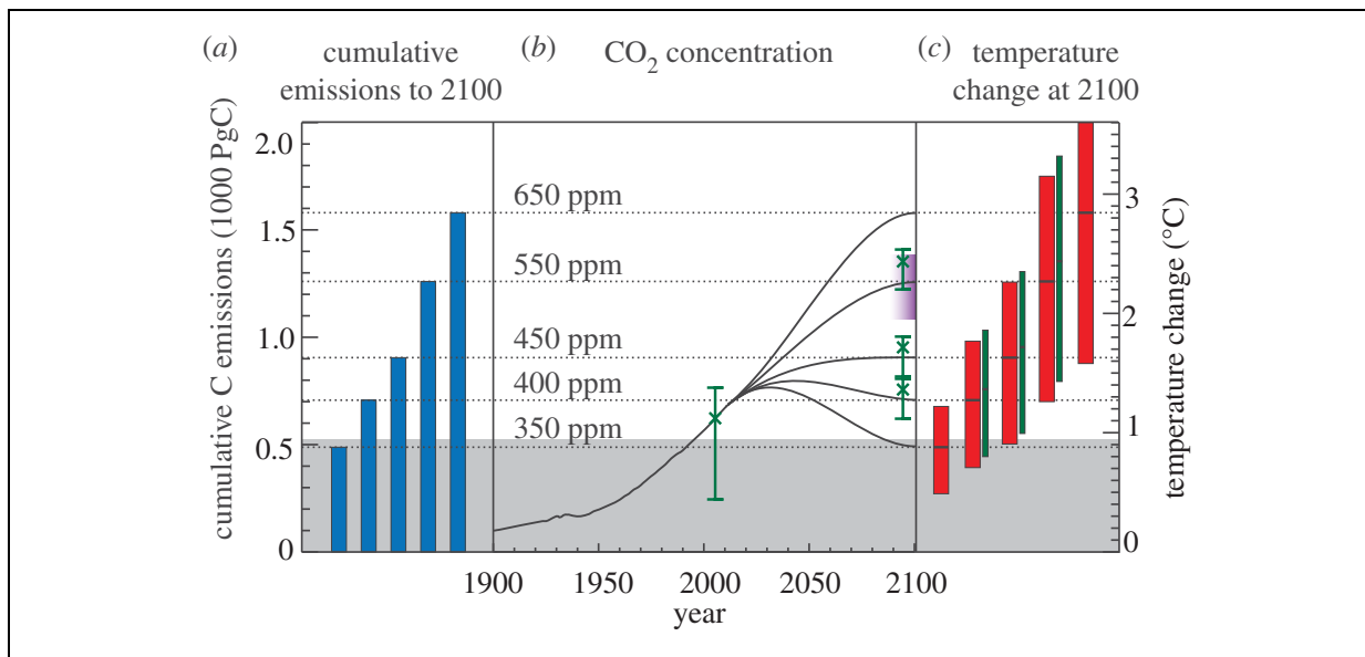
Figure 51 : Relation entre (a) les émissions cumulées en équivalent carbone, (b) les scénarios d'émissions de CO 2 et (c) l'élévation de la température globale à l'horizon 2100 (d'après le modèle numérique UVic ESCM)
