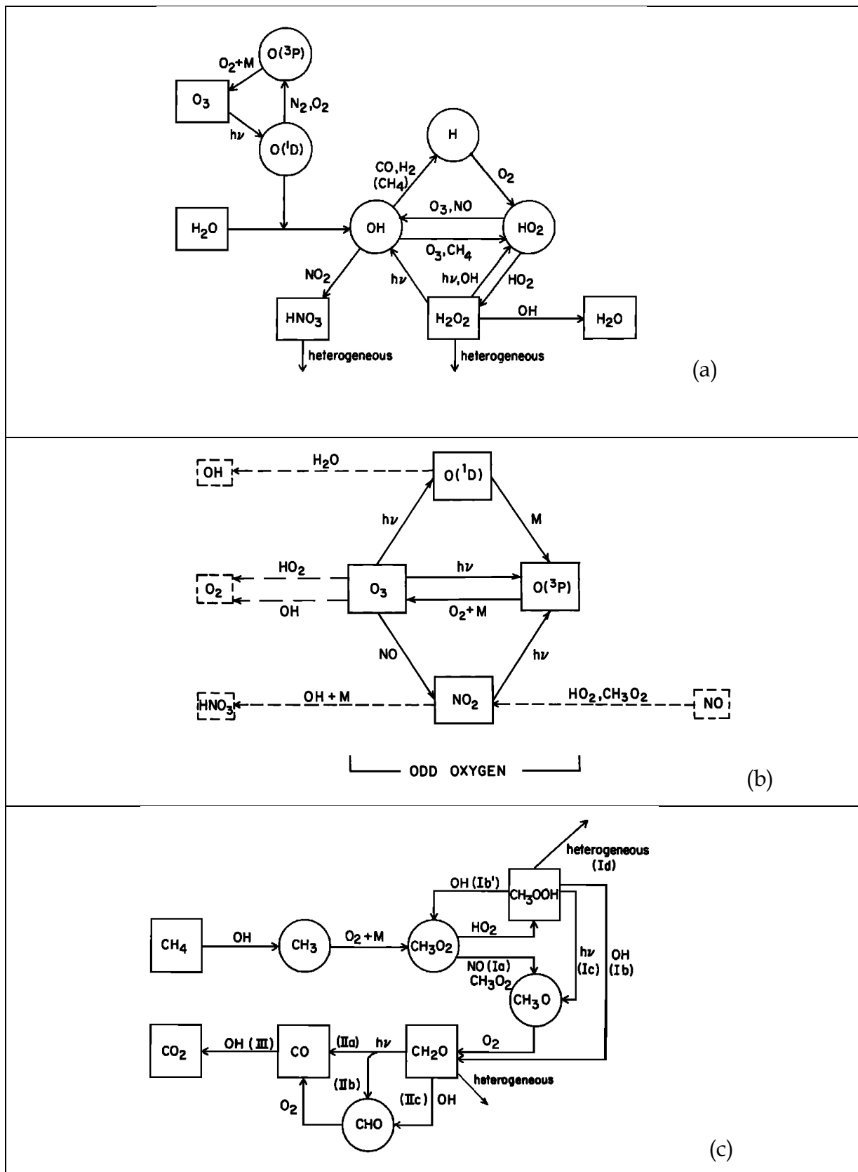
Figure 32 : Trois schèmes de réactions chimiques troposphériques aux implications globales [Logan et al. , 1981, pp. 7211, 7213 & 7216]
