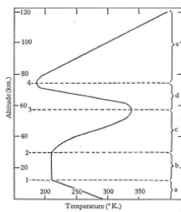
Figure 2 : Cinq nomenclatures atmosphériques, proposées au début des années 1950 par Goody (schéma et colonne de gauche), Flöhn et Penndorf, et Chapman [Goody, 1954, « Figure 2 : Approximate vertical temperature distribution in the atmosphere in temperate latitudes » & « Table I : Atmospheric nomenclature », pp. 5-6]
