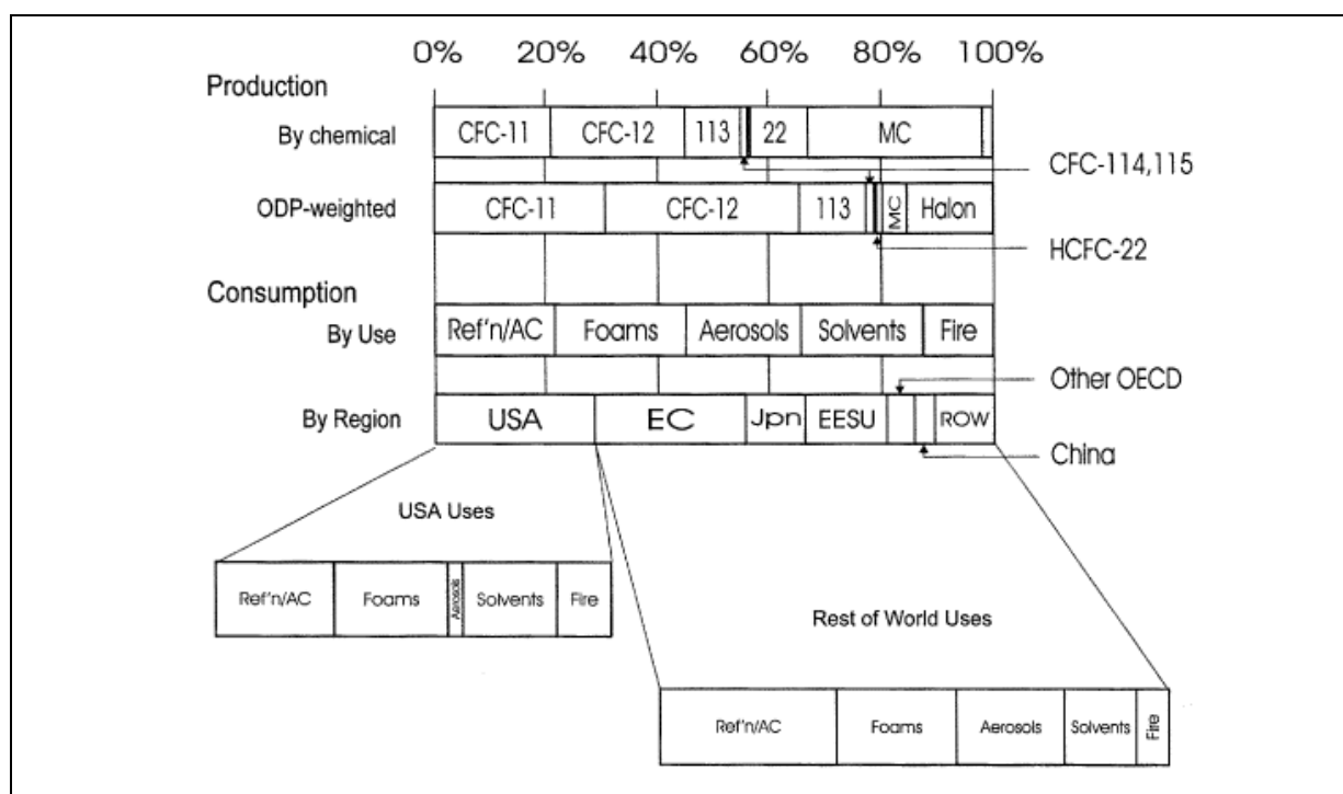
Figure 36 : Production et consommation des produits chimiques destructeurs d’ozone en 1986, dont la part de nocivité lié à la production des CFC-11, CFC-12, CFC-113, CFC-114 & -115, HCFC-22, méthylchloroforme (MC) et halons calculée d’après les valeurs de leurs ODP [Parson, 2003, “Figure 7.1”, p. 174, “Author’s calculations, based on Data from AFEAS 1995, Midgley 1989, EPA 1988, UNEP 1999 & UNEP 2002]
