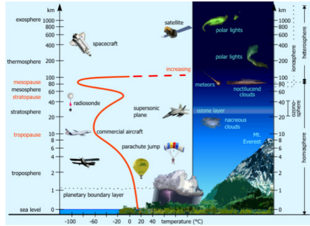
Figure 1 : Couches atmosphériques, phénomènes et procédés d’études de la haute atmosphère (a) en 1942 et (b) en 2011 (échelles d’altitudes logarithmiques) [Barbier & Chalonge, 1942, « Figure 5 », p. 36 ; http://www.theozonhole.com/atmosphere.htm (04/06/2011)]
