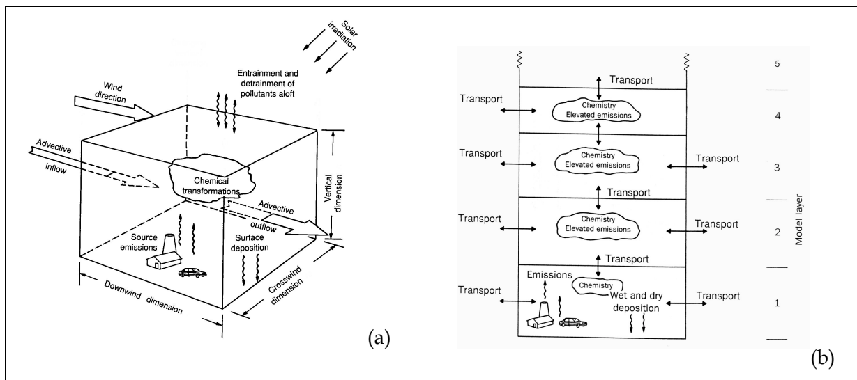
Figure 43 : Exemple de diagrammes schématiques de deux CTM eulériens, (a) l'un à zéro dimension, et (b) l'autre à une dimension (l'altitude) [ http://irina.eas.gatech.edu/ATOC3500_Fall1998/Lecture29.pdf (10/03/2014)]
