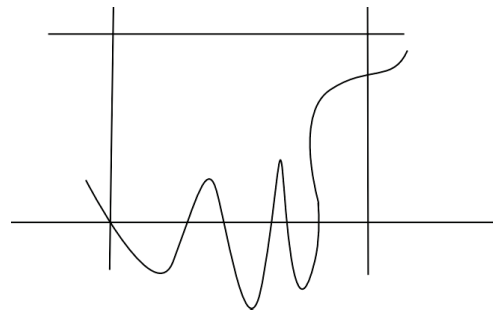
FIGURE 4.3.2 – Après une suite d'éclatement de points donnés par l'intersection de la courbe et L_\infty , suivi d'une suite de contraction, on obtient \mathbb{F}_d
