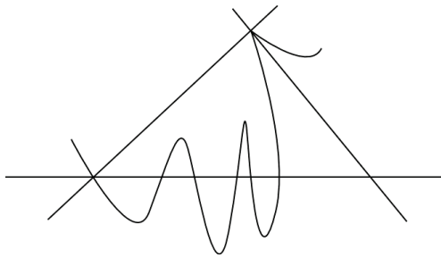
FIGURE 4.3.1 – Plongement dans \mathbb{P}^2
