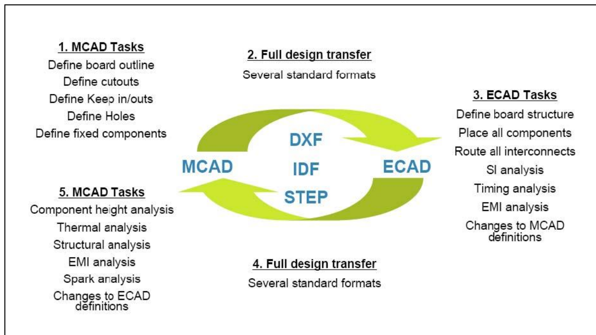
Figure 2.5 Procédure d'échange d'informations entre les métiers mécanique et électrique/électronique (Chen and Schaefer, 2007)
