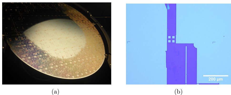
FIGURE 3.2 – Observations macroscopique (a) et microscopique (b) d'une plaque 300 mm avec motifs de résine sur TiN après traitement prolongé de SC1 et décolllement massif.
