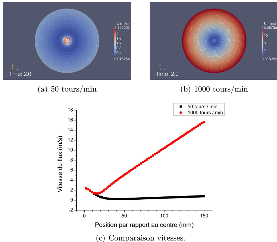
FIGURE 4.25 – Répartition de la valeur de célérité moyenne du fluide sur une plaque 300 mm en rotation à 50 tours/min (a) et 1000 tours/min (b). Comparaison sur un diamètre de la valeur de cette composante à chacune des vitesses de rotation (c)
