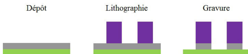
FIGURE 1.4 – Etapes successives permettant la structuration de l'empilement pour la réalisation des dispositifs en microélectronique.
