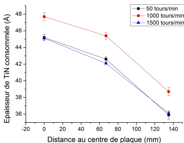
FIGURE 4.30 – Répartition de la quantité de TiN gravée par 120 s de SC1 sur une plaque de TiN en fonction de la vitesse de rotation de la plaque durant l'injection, mesurée par XRF.
