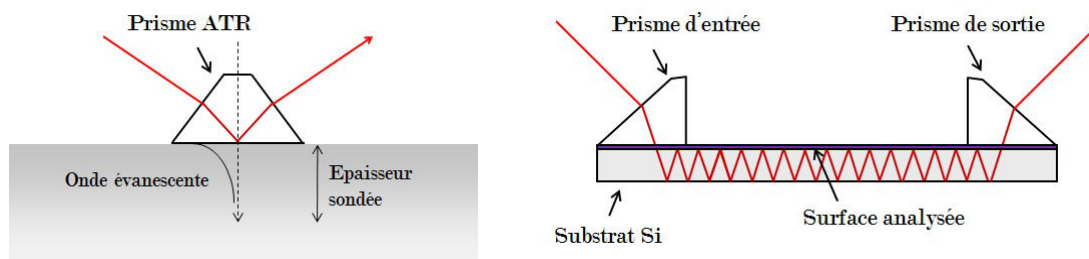
(a) Schéma d'un dispositif ATR "classique"
