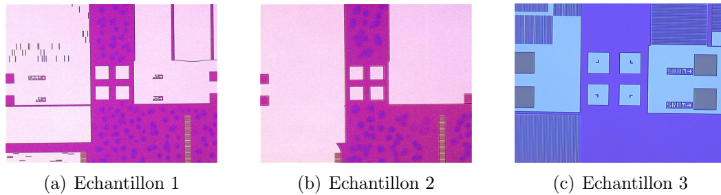
FIGURE 4.17 – Vue des motifs de résine de référence après traitement SC1 de 180 s sur les différents échantillons.
