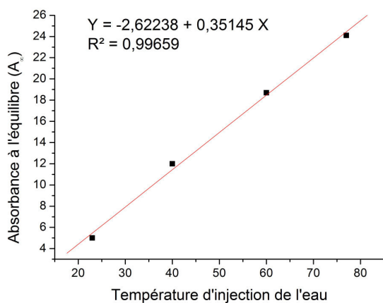
FIGURE 5.27 – Evolution de la valeur de A_\infty en fonction de la température d’injection de l’eau.
