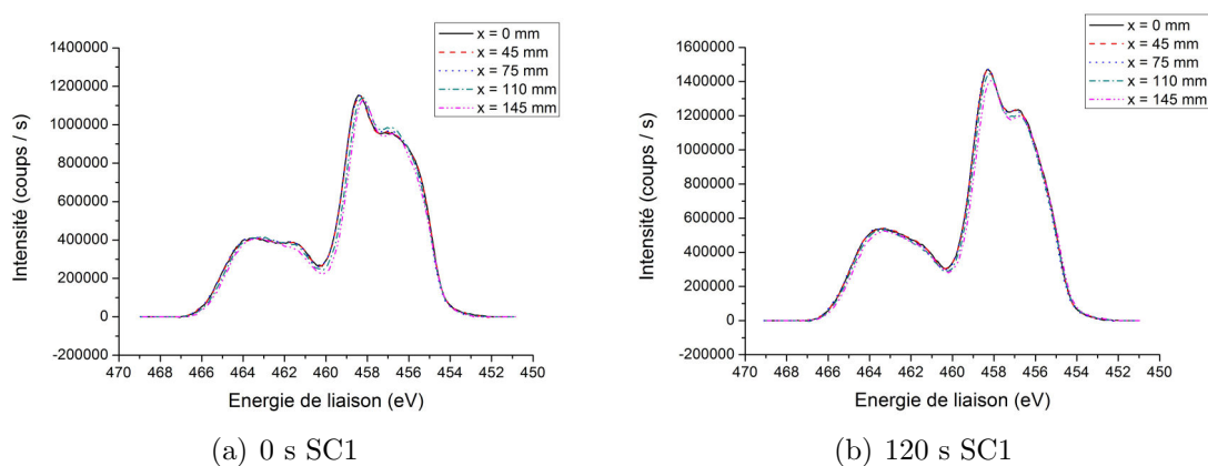
FIGURE 5.13 – Evolution du spectre XPS du Ti_{2p} en différents points de mesure répartis sur le rayon de la plaque 300 mm pour des échantillons sans traitement SC1 (a), et ayant reçu un traitement SC1 de 120 s (b).
