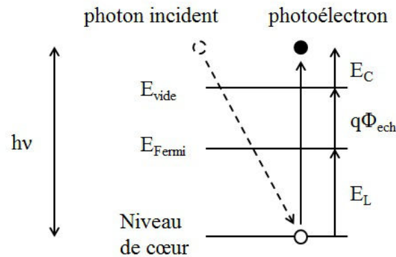
FIGURE 2.10 – Représentation schématique du phénomène d'émission de photoélectron et de conservation de l'énergie par effet photoélectrique.
