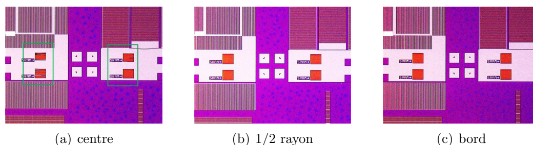
FIGURE 4.8 – Répartition spatiale en fonction de la position sur la plaque de la dégradation des motifs de résine sur TiN oxydé par plasma N_2 , après gravure chimique SC1 de 180 s.
