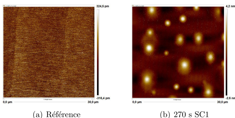
FIGURE 5.8 – Profils AFM des surfaces de résidu de résine post retrait plasma, pour une référence sans traitement chimique (a), et un échantillon ayant reçu un traitement SC1 de 270 s.
