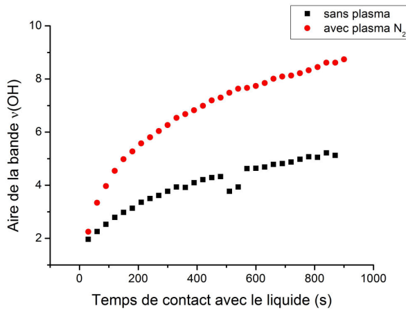
FIGURE 5.29 – Evolution de l'absorbance de la bande \nu(OH) en fonction du temps de contact avec l'eau pour des échantillons avec et sans plasma N_2 de nettoyage.
