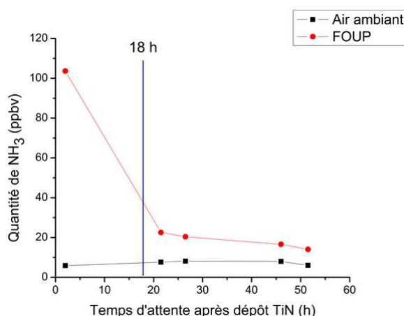
FIGURE 3.20 – Evolution de la concentration en NH_3 dans le FOUP en fonction du temps d'attente post dépôt du TiN.
