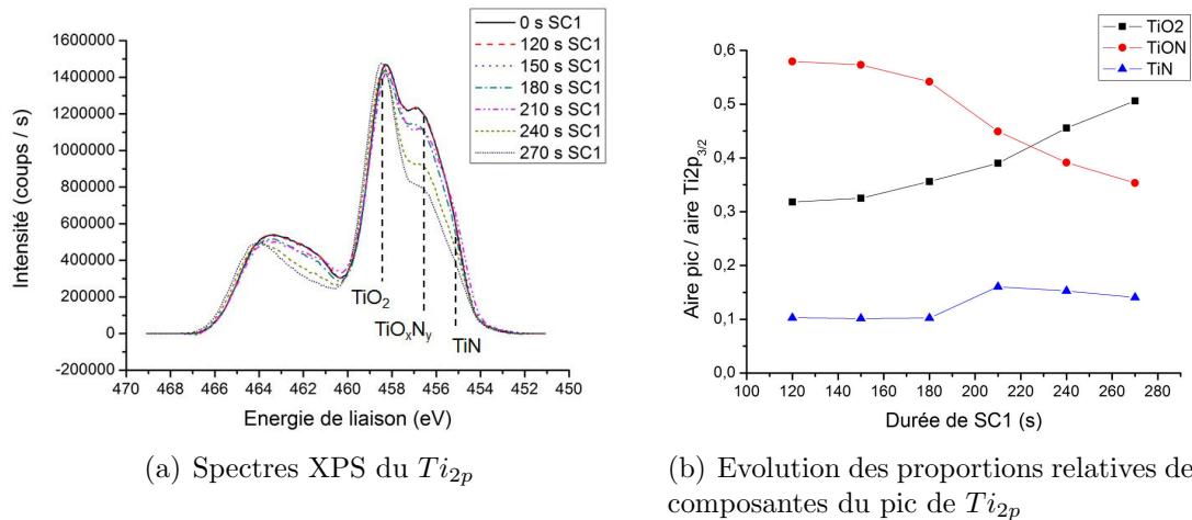
FIGURE 5.12 – Evolution du spectre XPS du Ti_{2p} pour différentes durées de traitement SC1 (a), et de la répartition en proportion des pics associés aux liaisons du titane (b) pour des points de mesure en centre de plaque
