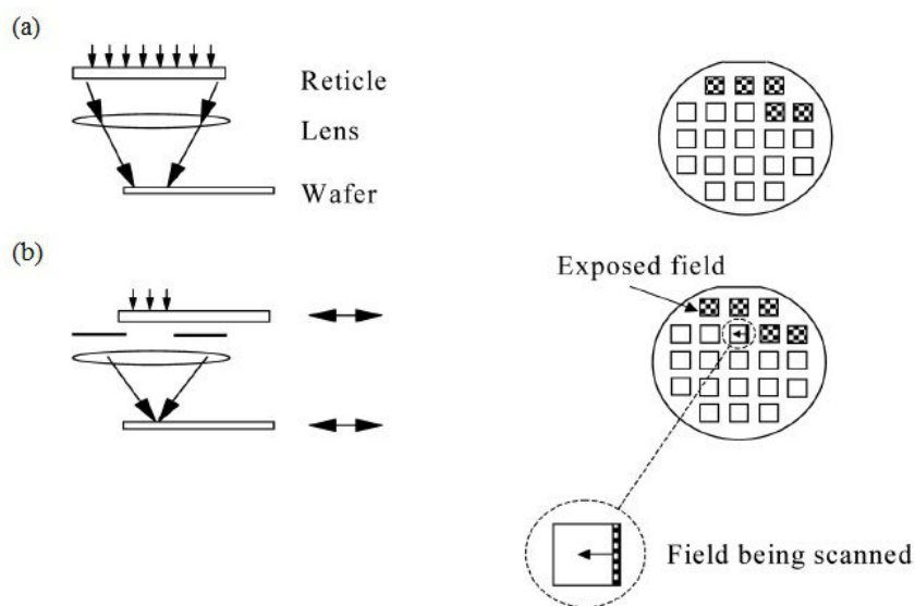
FIGURE 2.4 – Description des procédures d’exposition ”step-and-repeat”(a) et ”step-and-scan” (b) [44].
