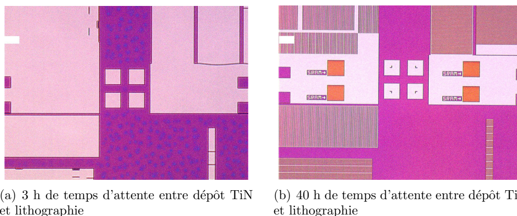
FIGURE 3.7 – Motifs de résine au centre de plaques ayant reçu un traitement chimique SC1 de 180 s avec un intervalle de (a) 3 h et (b) 40 h entre dépôt TiN et lithographie.
