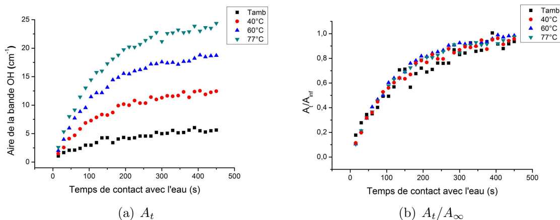
FIGURE 5.26 – Evolution de l’aire de la bande d’absorption \nu(OH) en fonction du temps de contact avec l’eau pour différentes températures d’injection, sans (a) et avec normalisation par rapport à la valeur d’absorbance à l’équilibre (b).
