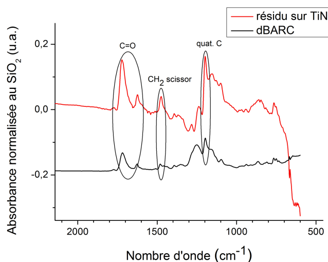
FIGURE 4.3 – Comparaison des spectres ATR de la couche organique résiduelle sur TiN (recuit à 190°C du dBARC) et de la référence de dBARC.
