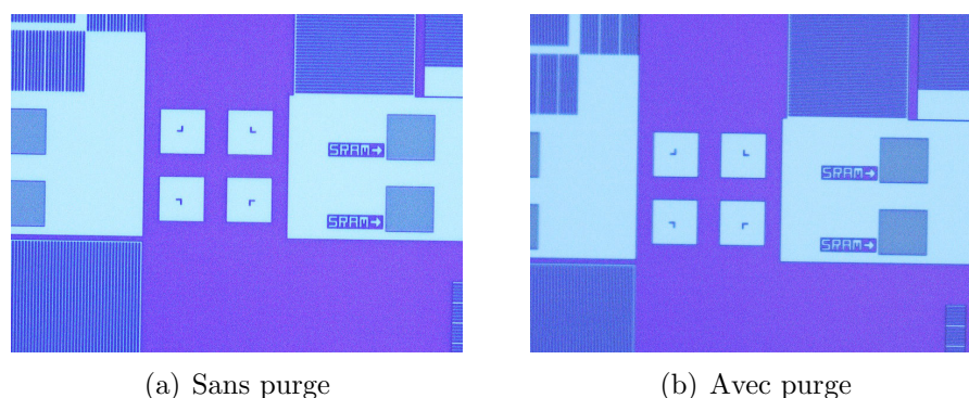
FIGURE 4.19 – Motifs de référence en centre de plaque après 210 s de gravure SC1 pour des plaques de TiN de référence (a) et ayant reçu un stockage en atmosphère inerte et des purges sous vide (b). Même intervalle de 48 h entre dépôt TiN et lithographie.
