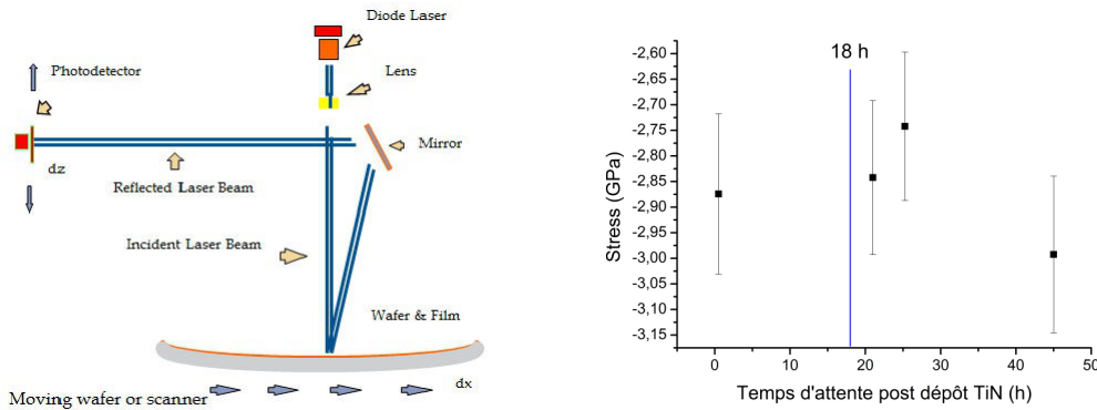
(a) Principe de fonctionnement de l'équipement de mesure du rayon de courbure.
