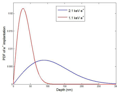
FIGURE 5.9 – Profils d'implantation du positronium à différentes énergies.
