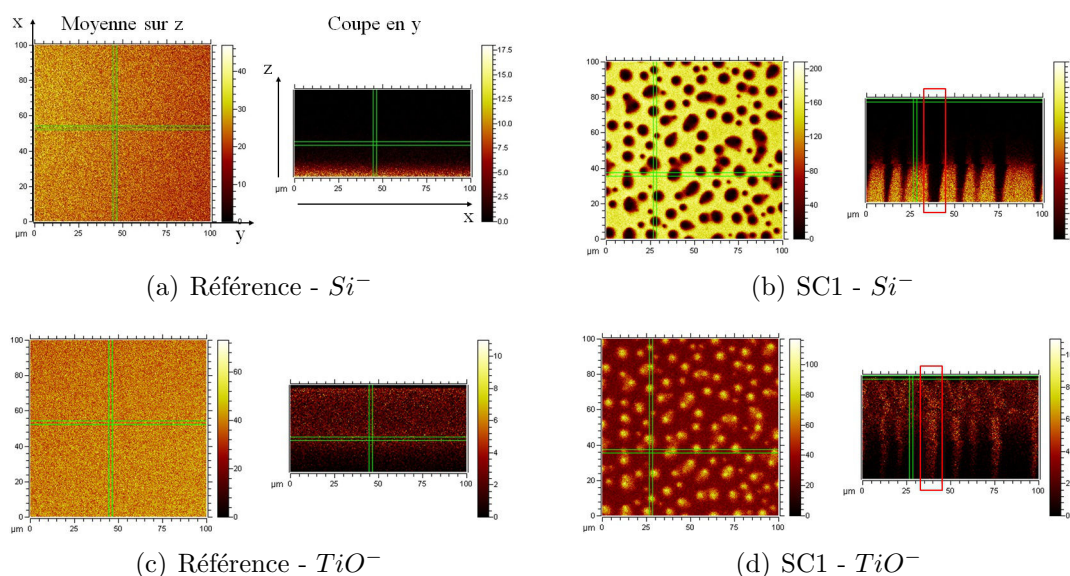
FIGURE 5.16 – Visualisations 3D et profils en épaisseur obtenus par ToF-SIMS pour les ions Si^- (a, b) et TiO^- (c, d) pour l'échantillon de référence (a, c) et celui ayant reçu un traitement SC1 de 270 s (b, d).
