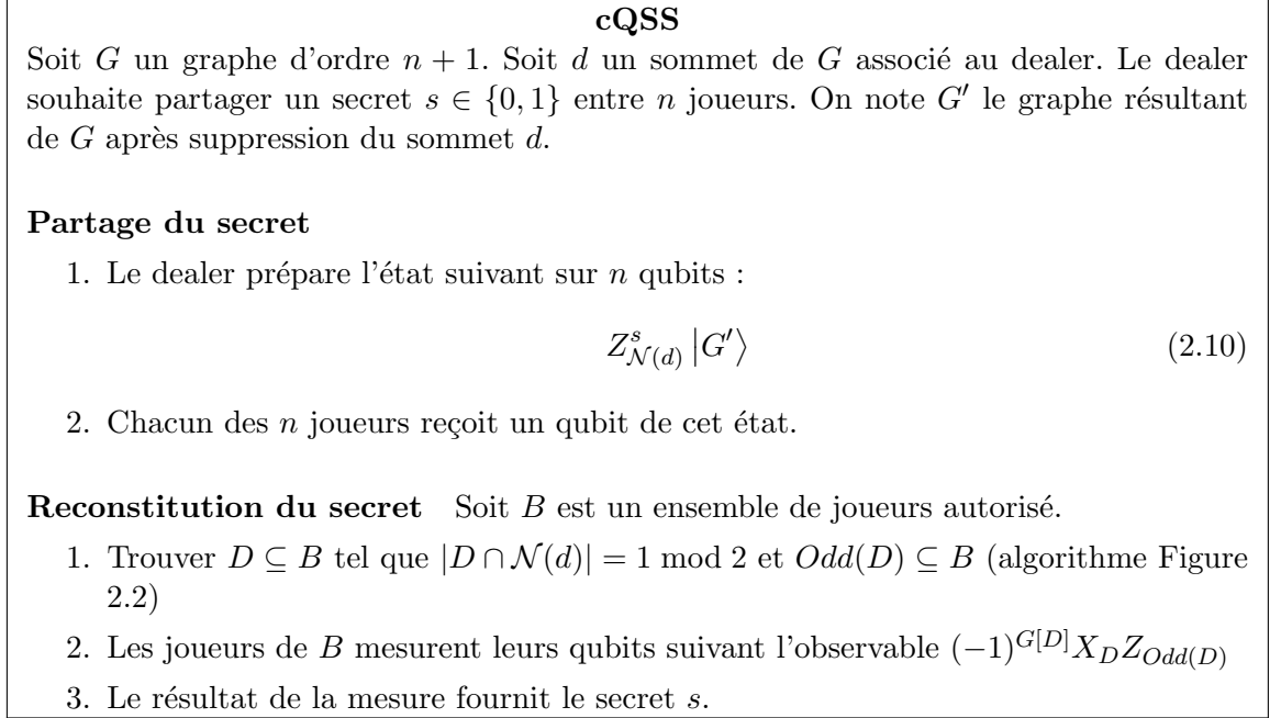
FIGURE 2.1 – Protocole de partage de secret classique avec des états graphes cQSS
