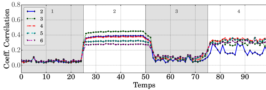
(a) Comparaison avec un réseau avec k communautés, pour différentes valeurs de k .
