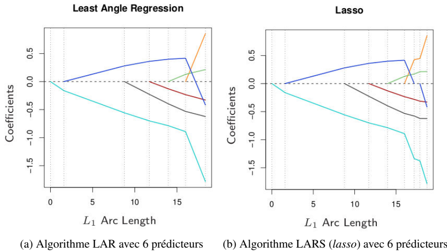
FIGURE A.7 – Évolution des coefficients à chaque étape pour 6 prédicteurs. (a) Algorithme LAR. (b) Algorithme LARS ( lasso ). [98]
