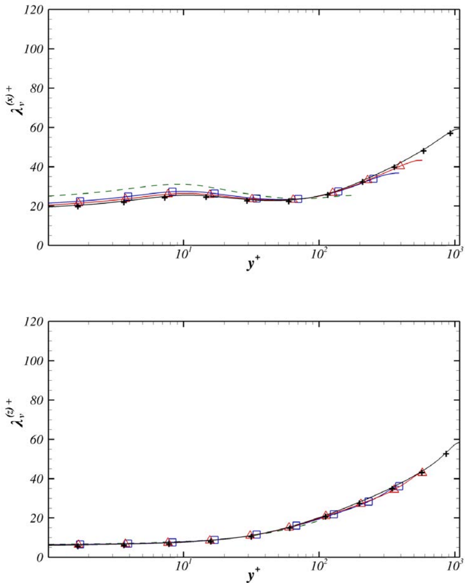
FIGURE 9.4 – Échelles de Taylor associées aux fluctuations de vitesse normale dans les directions longitudinale et transverse pour Re_\tau = 180, 395, 590 et 1100 .
