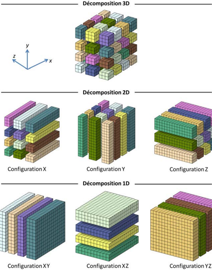
FIGURE 1.2 – Décomposition 1D, 2D et 3D du domaine de calcul
