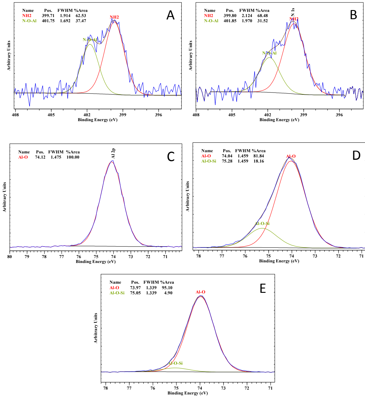
Figure 2.6.4. Spectres du niveau d'énergie N\ 1s pour APS-01 (7% H_1 T_{30\text{ min}}^{40^\circ\text{C}} Ba) (A), APS-04 (3.5% H_1 T_{30\text{ min}}^{40^\circ\text{C}} Ba) (B) et spectre du niveau Al\ 2p pour APS-01 (7% H_1 T_{30\text{ min}}^{40^\circ\text{C}} Ba) (C), APS-04 (3.5% H_1 T_{30\text{ min}}^{40^\circ\text{C}} Ba) (D) et de la boehmite pure (E)
