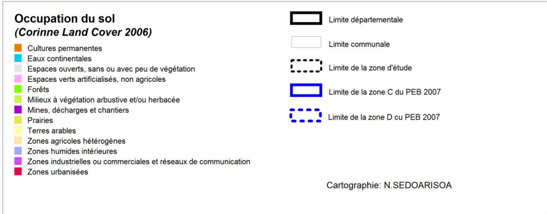
Figure 6: Occupation du sol autour de l'aéroport de Toulouse-Blagnac
