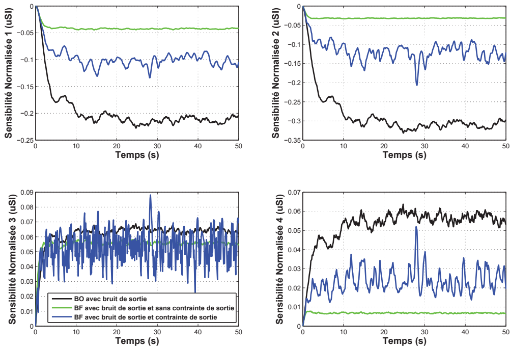
FIGURE 5.17 – RCPC avec bruit : sensibilités normalisés des états du modèle par rapport aux paramètres inconnus.
