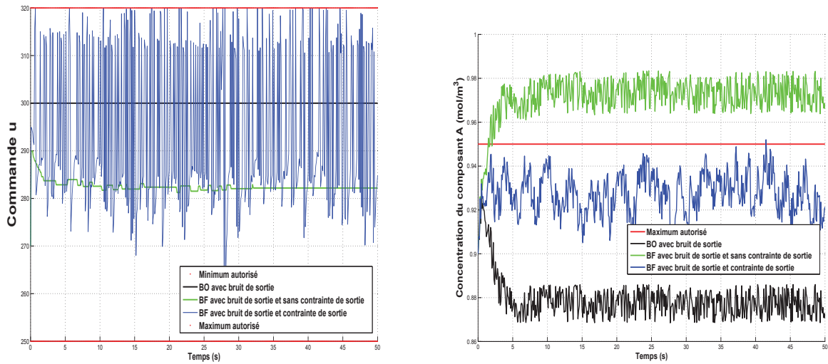
(a) u : la température de l'enveloppe de refroidissement, T_c . (b) y_{p1} : la concentration du composant A.
