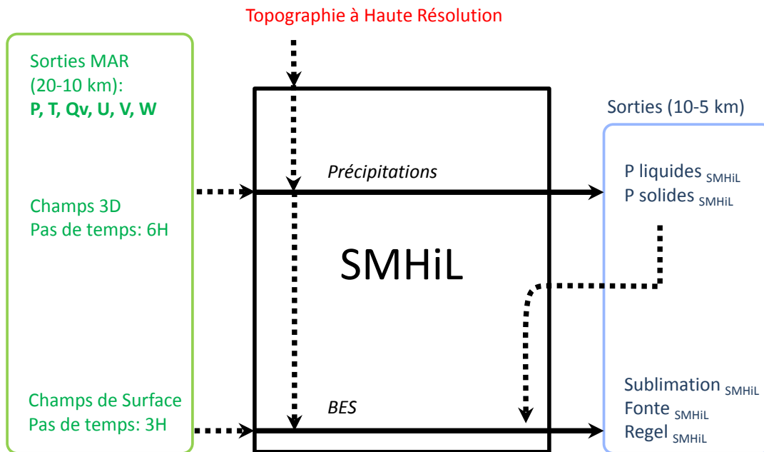
FIGURE 2.11 – Schéma décrivant le fonctionnement du modèle SMHiL. D'après une présentation de Cécile Agosta (2012).
