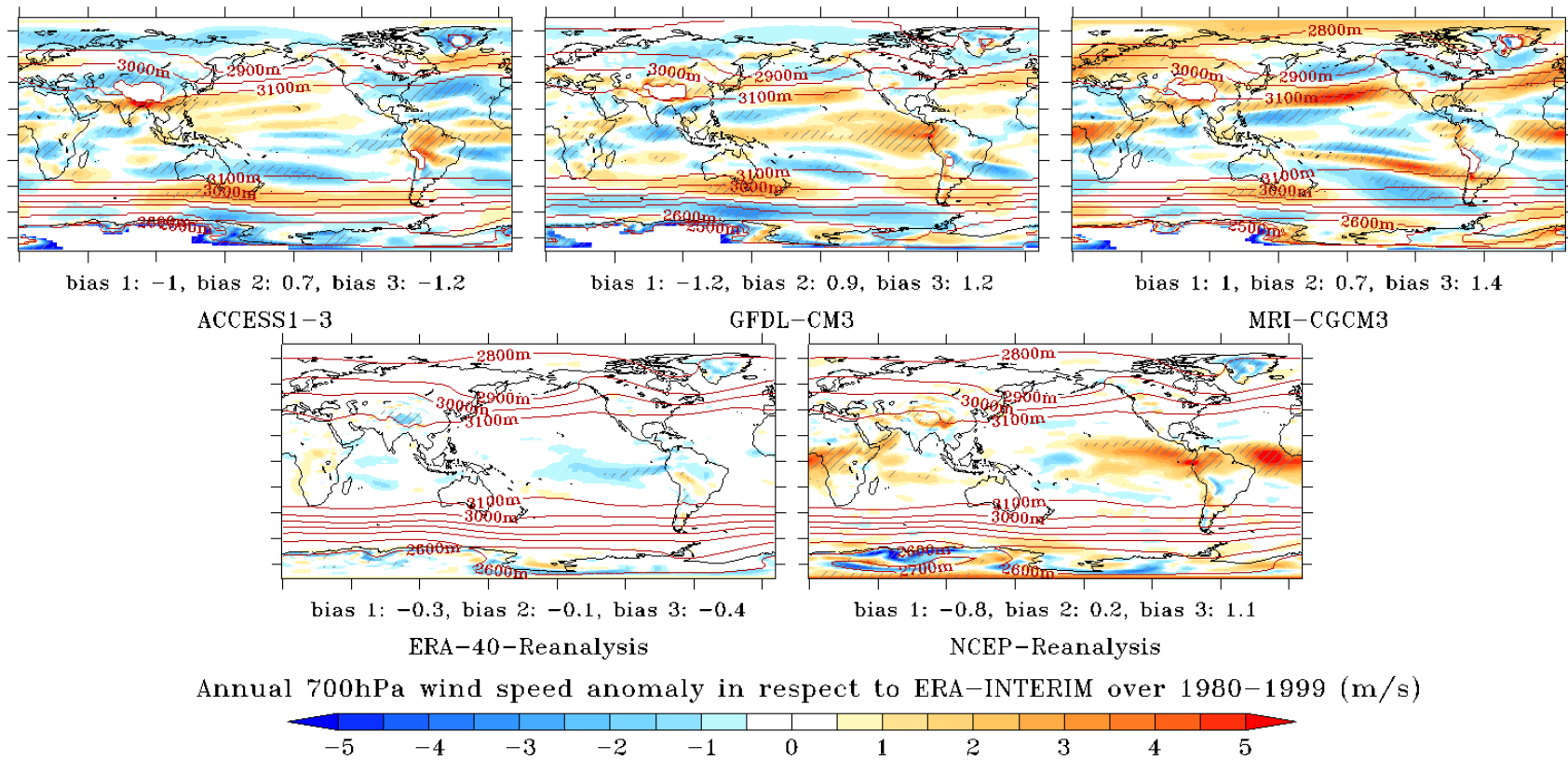
FIGURE 3.3 – Anomalie moyenne ( \overline{WS}_{CMIP5} - \overline{WS}_{ERA-Int} ) de vitesse du vent annuelle à 700hPa par rapport à ERA-Interim sur la période 1980-1999, tracée sur la grille d'ERA-Interim, pour ACCESS1-3, GFDL-CM3, MRI-CGCM3, ERA-40 et NCEP1. Les biais indiqués sont calculés de la manière suivante : (\overline{WS}_{CMIP5} - \overline{WS}_{ERA-Int})/\sigma(WS_{ERA-Int}) , où \sigma représente l'écart-type. Le biais 1 est calculé sur l'ensemble de la zone 40° S - 90° S, le biais 2 sur la zone 40° S - 60° S et le biais 3 sur la zone 60° S - 90° S. Les contours correspondent à la hauteur du géopotiel 700 hPa. Les zones hachurées représentent les endroits où l'anomalie de vitesse du vent est plus de deux fois supérieure à l'écart-type de la vitesse du vent dans le modèle CMIP5.
