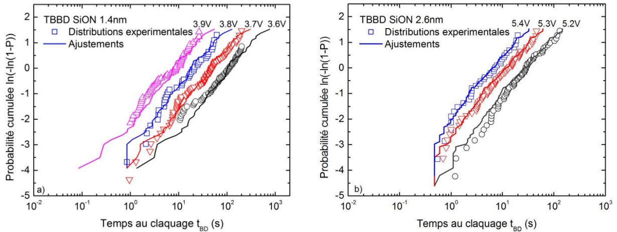
Figure 5.13 : Distributions cumulées TDDB obtenues par C-AFM sur SiON 1,4nm pour quatre tensions de stress différentes (a) et sur SiON 2,6nm pour trois tensions de stress différentes (b) et reproduites par simulation Monte-Carlo avec 150 tests en utilisant les paramètres du tableau 5.2.
