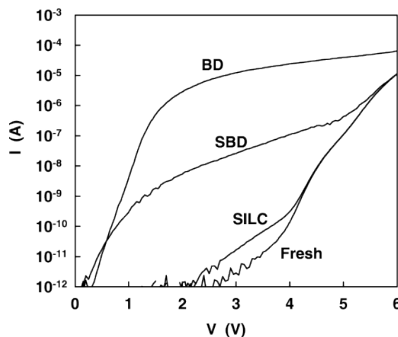
Figure 1.13 : Caractéristiques I(V) mesurées à différents états de rupture diélectrique. La courbe notée « Fresh » est obtenue lors de la première mesure sur un oxyde SiO_2 , la courbe SILC est obtenue après une contrainte non destructive, SBD et BD respectivement obtenues après observation d'un soft breakdown et hard breakdown [19].
