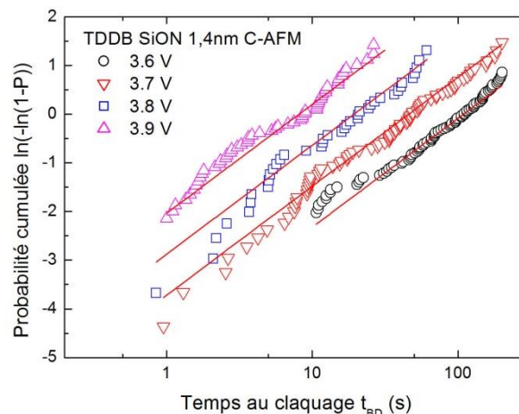
Figure 3.5 : Distributions des t_{BD} obtenues par C-AFM sur la couche IL de 1,4nm pour quatre tensions de grille (3,6-3,9V). Les distributions ont été ajustées avec l'équation (1.22) en utilisant le modèle en puissance (courbe rouge).
