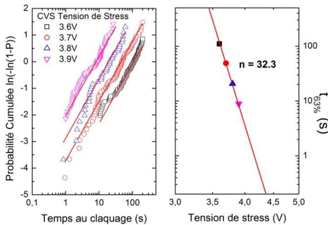
Figure 4.12 : Distributions cumulées des TDDB pour quatre tensions de stress différentes (Chapitre 3) (a). Valeurs de t_{63\%} extraites en fonction des tensions de stress. La courbe rouge est l'ajustement des données expérimentales suivant \log(t_{63\%}) = \text{const} - n \cdot \log(V) (b).
