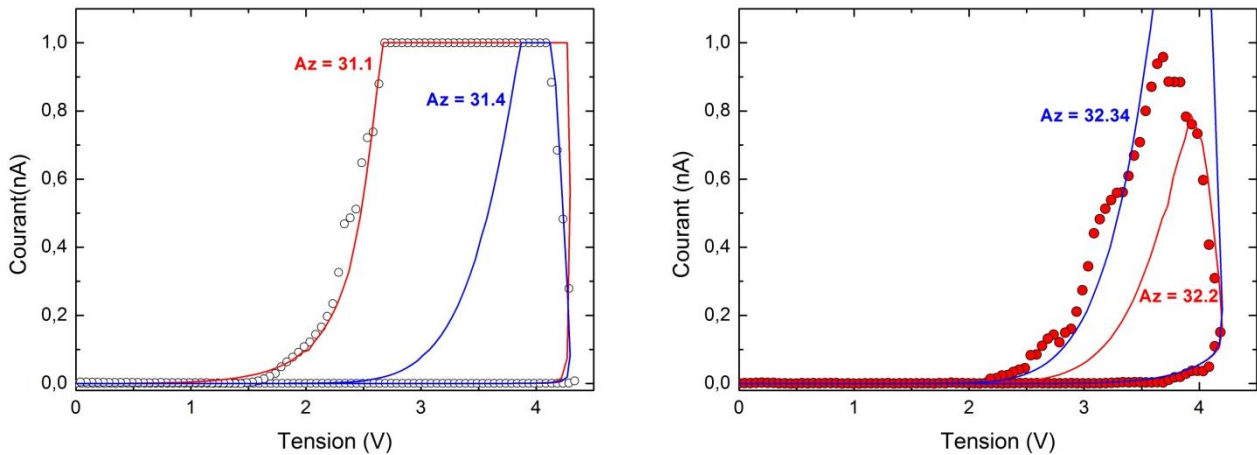
Figure 6.10: Ajustement des caractéristiques NDR obtenues avec TiN (a) et Ti (b) comme électrode inférieure à l'aide du modèle filamenteux présenté dans le chapitre 5. Aucune valeur de Az ne permet de reproduire à la fois la croissance et la décroissance du courant.
