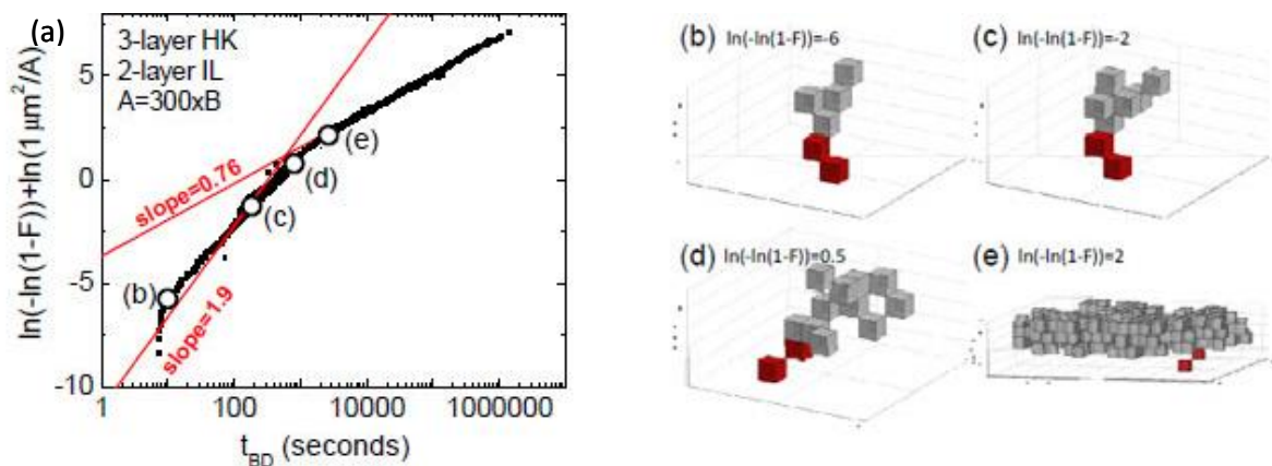
Figure 1.30 : Distributions simulées des TDDB obtenues par la méthode kMC sur un empilement constitué d'une couche High-k d'une épaisseur de trois cubes et d'une couche IL (a) d'une épaisseur de deux cubes. Défauts créés dans les couches au moment du claquage (b-e) [49].
