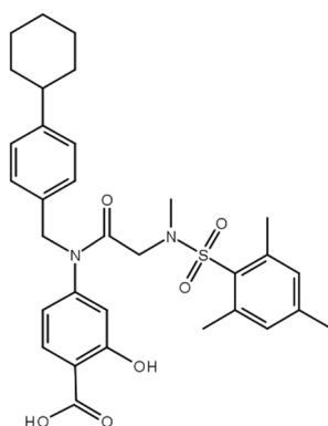
Figure 10: Structure chimique du BP-1-108.
