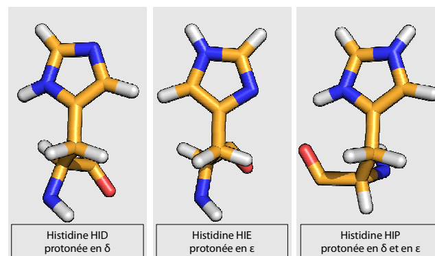
Figure 24 : Les différents états de protonation du résidu d'histidine.
