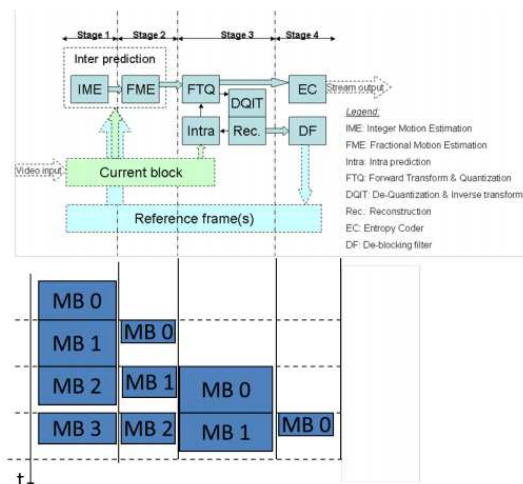
Figure 2: Architecture de pipeline classique d'un encodeur H.264 encodeur matériel.
