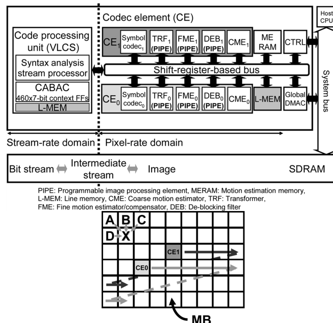
Figure 3: Encodeur H.264 orienté vitesse [Iwat09A].
