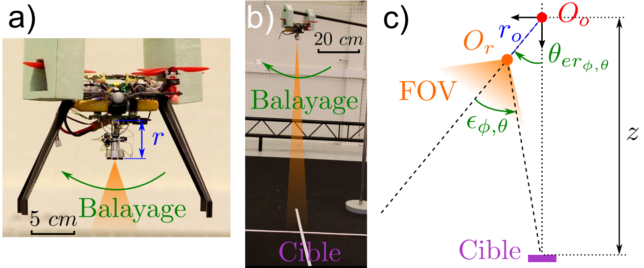
FIGURE IV.25 – a) Zoom sur le robot et son œil lors du processus de calibration des paires de photodiodes. b) Le robot est suspendu au dessus de la cible qui est placée à la verticale en dessous du robot. Ici z = 1.32 m. L'œil effectue un balayage latéral permettant de faire parcourir à la cible tout le champ visuel de l'œil. c) Représentation schématique des différentes grandeurs permettant de remonter à la relation géométrique entre l'orientation de l'œil \theta_{er_\phi} ou \theta_{er_\theta} et la position de la cible \Psi_{c_\phi} ou \Psi_{c_\theta} dans le champ visuel de l'œil.
