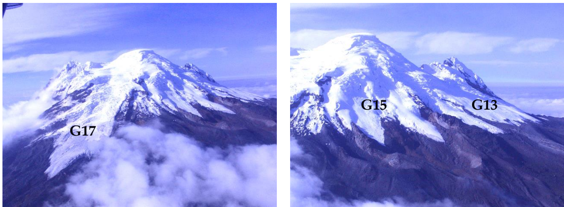
Figure 6.7. Glaciers du groupe I orientés vers l'ouest : la photo à gauche montre le glacier Antisana 17. La photo à droite montre les glaciers Antisana 15 et 13. Photos Patricia Mothes, 21 mai 2011.
