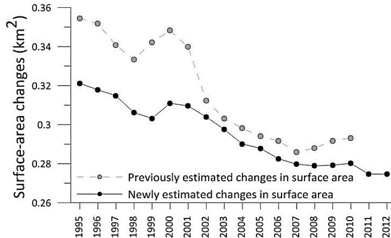
Figure 3.12. Comparaison de la variation de la surface du Glacier Antisana 15 \alpha : avec la limite déterminée par la cartographie IGM et les données géodesiques annuelles (cercles et ligne grise pointillée) et avec l'ajustement de la surface avec la nouvelle cartographie et les données géodesiques annuelles (cercles et ligne noire).
