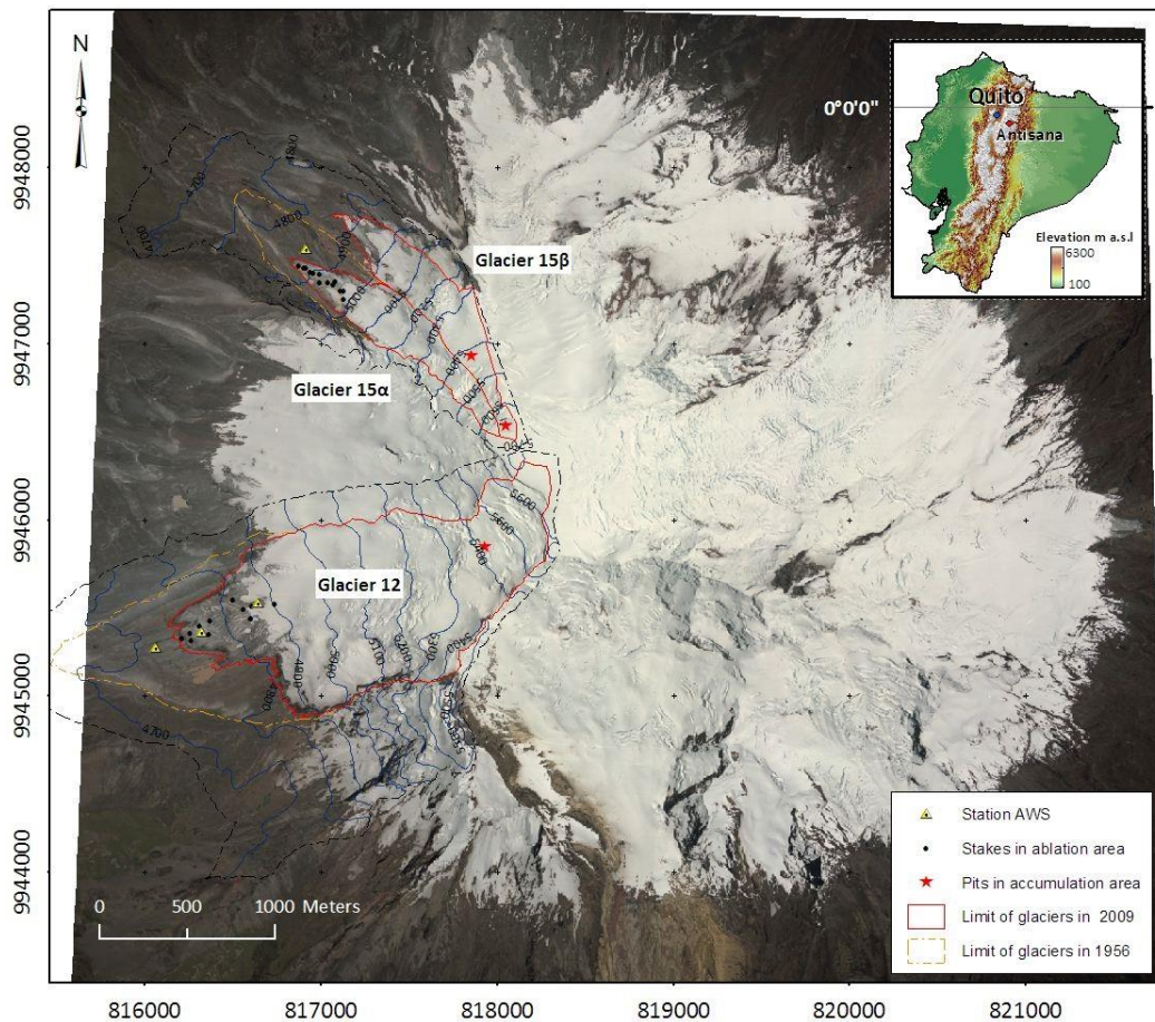
Figure 2.3. Localisation des glaciers Antisana 12 « Los Crespos » et Antisana 15. Le contour rouge continu et le contour orange pointillée montrent la limite des glaciers en septembre 2009 et février 1956 respectivement. La ligne noire pointillée est la surface restituée par photogrammétrie. Les points noirs représentent les balises dans la zone d'ablation, l'étoile rouge est le site de mesure d'accumulation et les triangles jaunes sont les stations météorologiques. L'insertion cartographique en haut et à droite présente la localisation du volcan Antisana (losange rouge) à 40 km à l'est de la ville de Quito, capitale de l'Équateur (losange bleu). Ortho-photo de 2009. UTM zone 17S, WGS84 (équidistance des courbes de niveau = 100 m).
