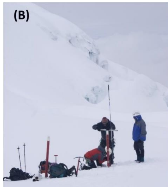
Figure 3.2. (A) Mesure mensuelle d'émergence des balises d'ablation. (B) Mesure annuelle d'accumulation. (Photos : B. Francou)
