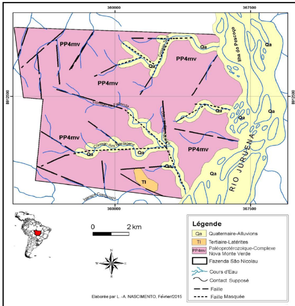
Figure 4.7. Carte géologique de la Fazenda São Nicolau, où affleurent les roches appartenant au Complexe Nova Monte Verde (Modifiée à partir des données de la CPRM, 2004a, 2011 ; l'IBGE, 2009 et SEPLAN 2011).
