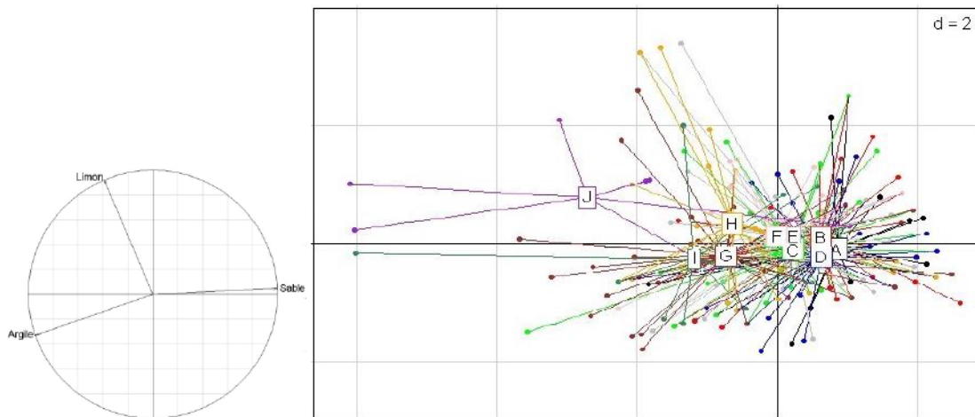
Figure 8.3. Les corrélations texture / classes de stockage de carbone. a : le cercle de corrélation (plan 1–2) ; b : la S-class entre les classes de carbone et les textures des sols.
