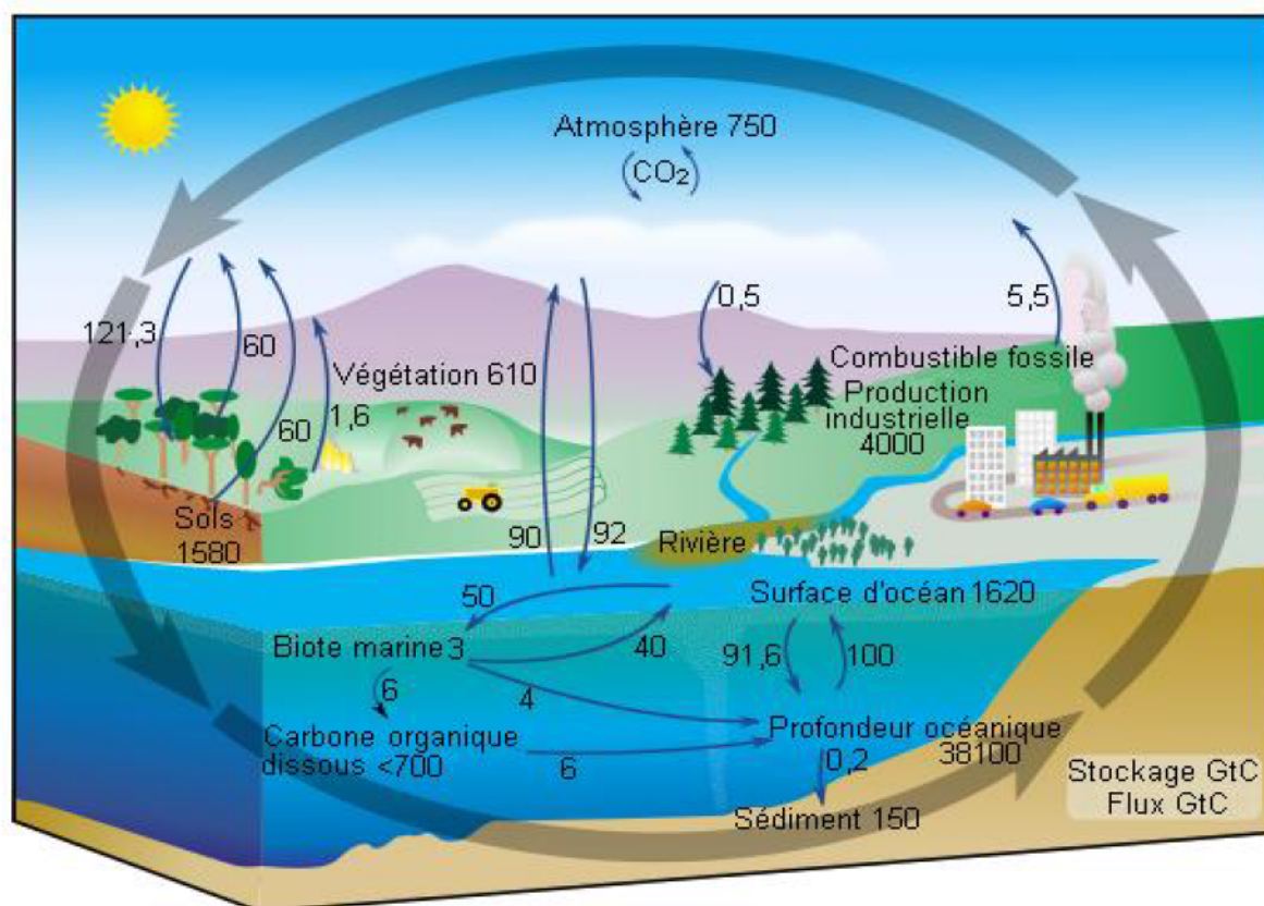
Figure 1.1. Esquisse du Cycle du Carbone (d'après Harrison in IPCC– Intergovernmental Panel Climate Change, 2003).
