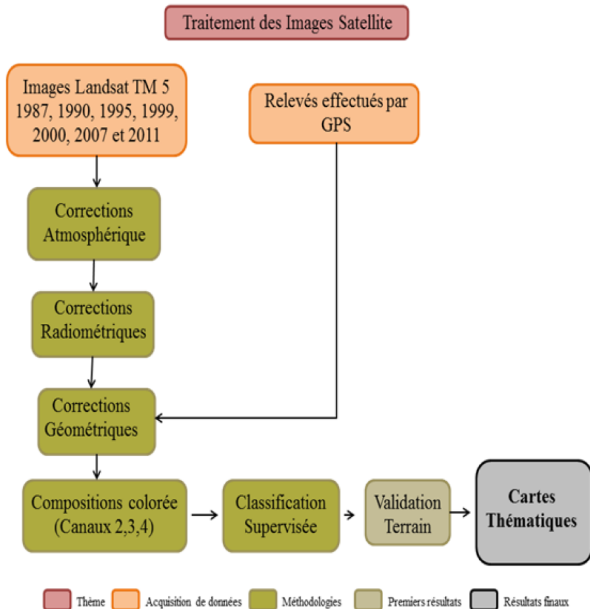
Figure 3.3. Organigramme du traitement des images satellitaires.
