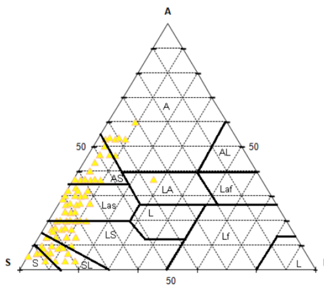
Figure 7.1. La texture des sols de la Fazenda São Nicolau (D'après le diagramme de texture de l'USDA 1960).
