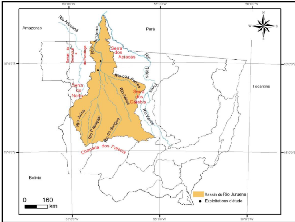
Figure 4.1. Bassin du Rio Juruena à l'Etat de Mato Grosso (Elaborée par L.-A. Nascimento, mai/2015).
