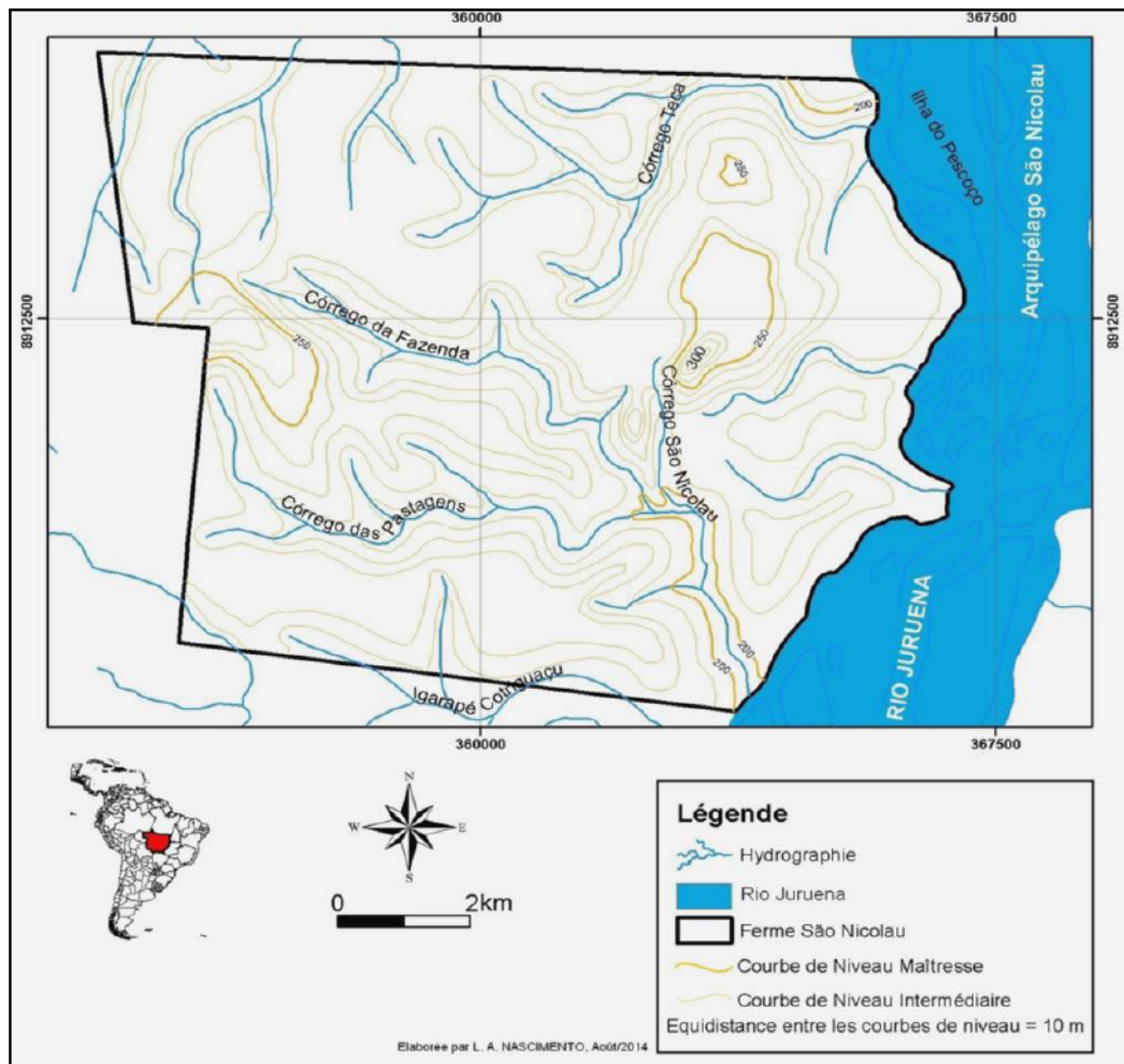
Figure 4.5. Carte hydrographique de la Fazenda São Nicolau. Nous pouvons remarquer aussi, dans le lit du Rio Juruena, une partie de l'Archipel São Nicolau (L.-A Nascimento, 2014).
