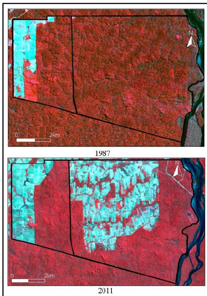
Figure 5.3. Comparaison entre les images de satellite Landsat TM 5 de 1987 et 2011 (CC 432) sur la Fazenda Preciosa et l'Assentamento Vale do Amanhecer (L.-A. Nascimento, septembre 2014).
