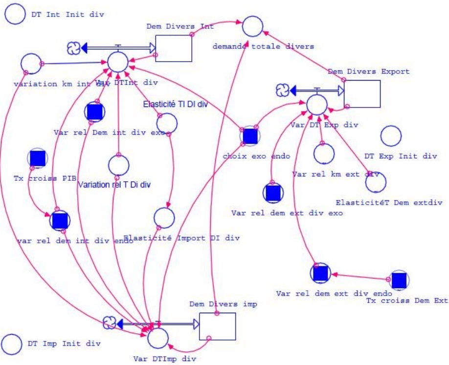
Figure 58: Exemple de bloc de calcul d'une demande sectorielle : le cas des produits divers
