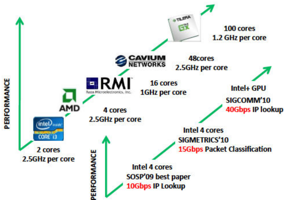
Figure 2 : Architecture Multi-cœurs et performances des routeurs logiciel
