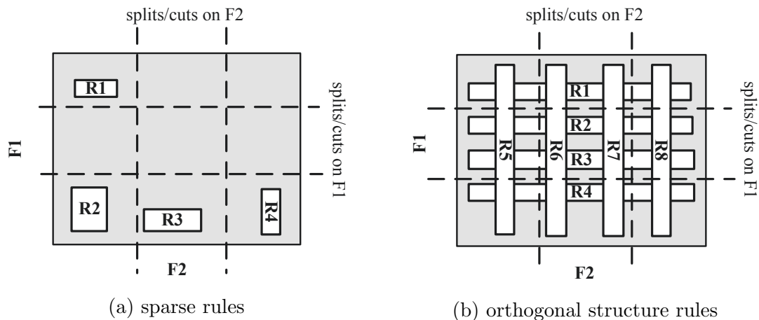
Figure 7- Structures orthogonales et règles clairsemées
