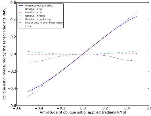
(a) Oblique astig. measurement
