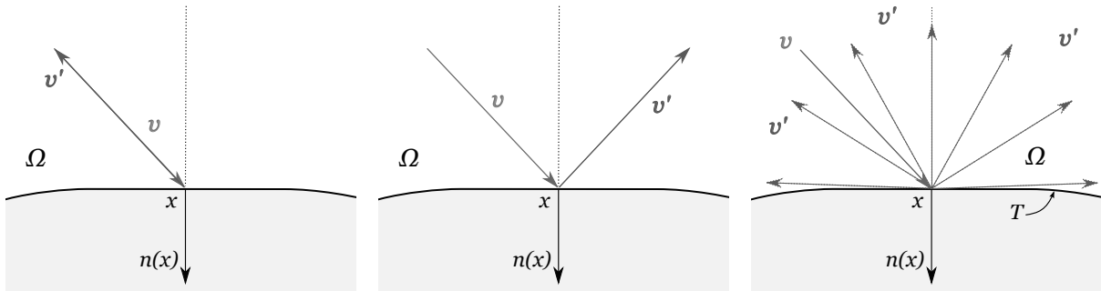
FIGURE 3.1 – Réflexion inverse FIGURE 3.2 – Réflexion spéculaire FIGURE 3.3 – Réflexion diffusive
