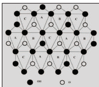
Figure 3 : Projection d'une couche octaédrique idéale d'un minéral de type 1/1 montrant la position des atomes d'oxygène et des groupements hydroxyles des différents sites octaédriques (Drists et Tchoubar, 1990)
