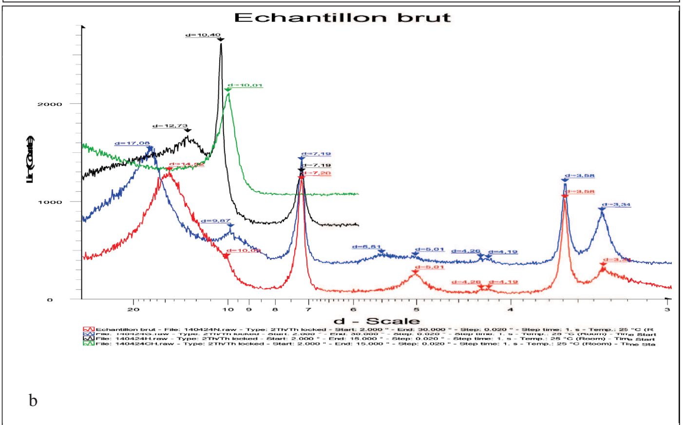
Figure 9 : Diffractogrammes des rayons X de l'argile de Fouchana (a : fraction totale ; b : fraction < 2 μm)
