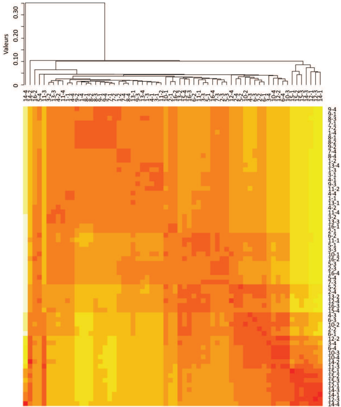
Figure 15: Classification hiérarchique basée sur la distance euclidienne et carte de chaleur associée obtenues sur les métriques de l'I2M2 calculées pour le substrat racines sur la Vienne (carte de chaleur : rouge = proche, blanc = complètement différent ; le premier numéro = code laboratoire, 16 laboratoires, et le deuxième = code répétition, 4 répétitions de substrats, exemple : laboratoire 10 – répétition 3)
