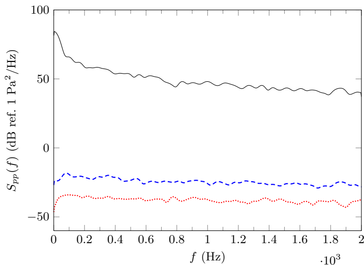
FIG. 2.20 – DSP des composantes aérodynamique (---) et acoustique ( \cdots ); des pressions reconstruites par RI (—) à partir du champ de déplacement bruité (RSB = 40 dB).
