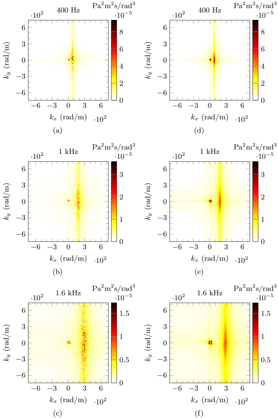
FIG. 2.4 – Spectres en fréquence-nombre d'onde S_{pp'}(k_x, k_y, \omega) des signaux temporels synthétisés et correspondant à la somme du modèle de Corcos et d'un champ diffusif acoustique pour 3 fréquences différentes : (a) 400 Hz, (b) 1 kHz et (c) 1.6 kHz. Les spectres théoriques sont représentés pour les mêmes fréquences respectivement en (d), (e) et (f).
