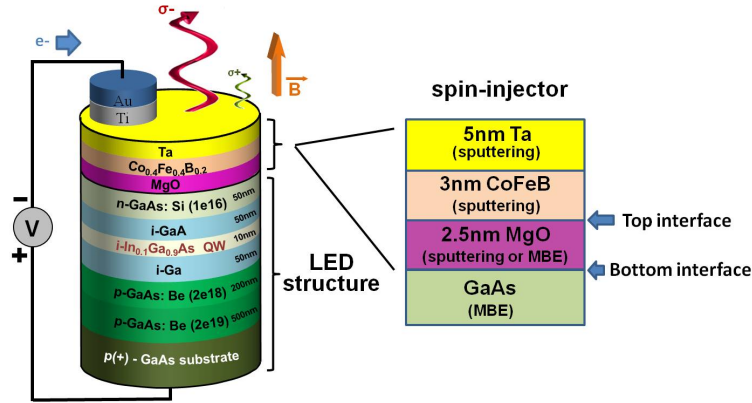
Figure 3: Schéma de principe d'une Spin-LED.
