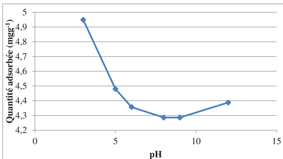
Figure 4.4: effet du pH sur l'adsorption du FB par l'argile de Borj Chekir
