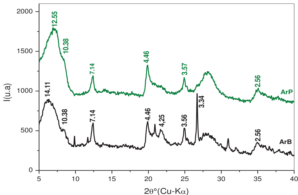
Figure 3.3 Diffractogrammes de RX des échantillons brut et purifié de l'argile de Gafsa
