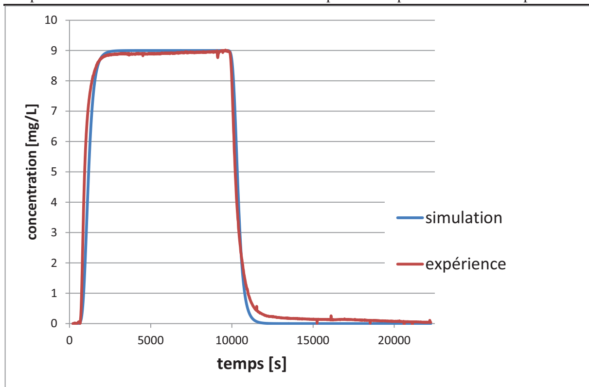
Figure 5.10 : Essai de traçage « mélange sable/argile à 30% » : courbes de sortie observées et simulées avec les paramètres calibrés ( n_{c,m}=0,02 , \alpha_{L,ch}=0,001 m)
