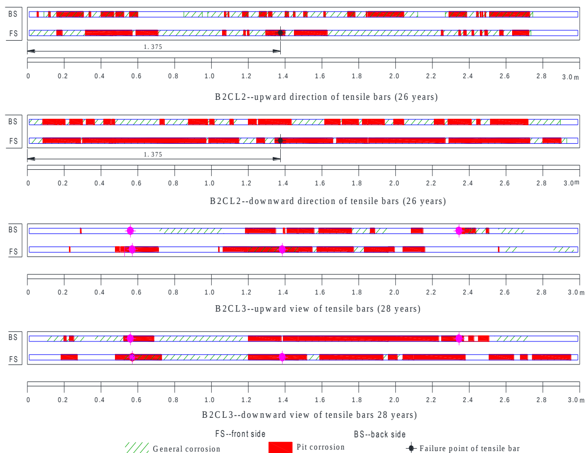
Figure 6: corrosion sur les barres longitudinales tendues
